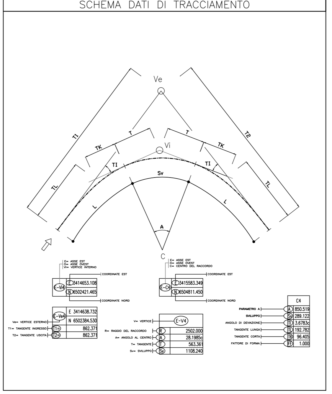
PLANIMETRIA DI PROGETTO E TRACCIAMENTO ADEGUAMENTO VIABILITA' ESISTENTE - SCALA 1:500
