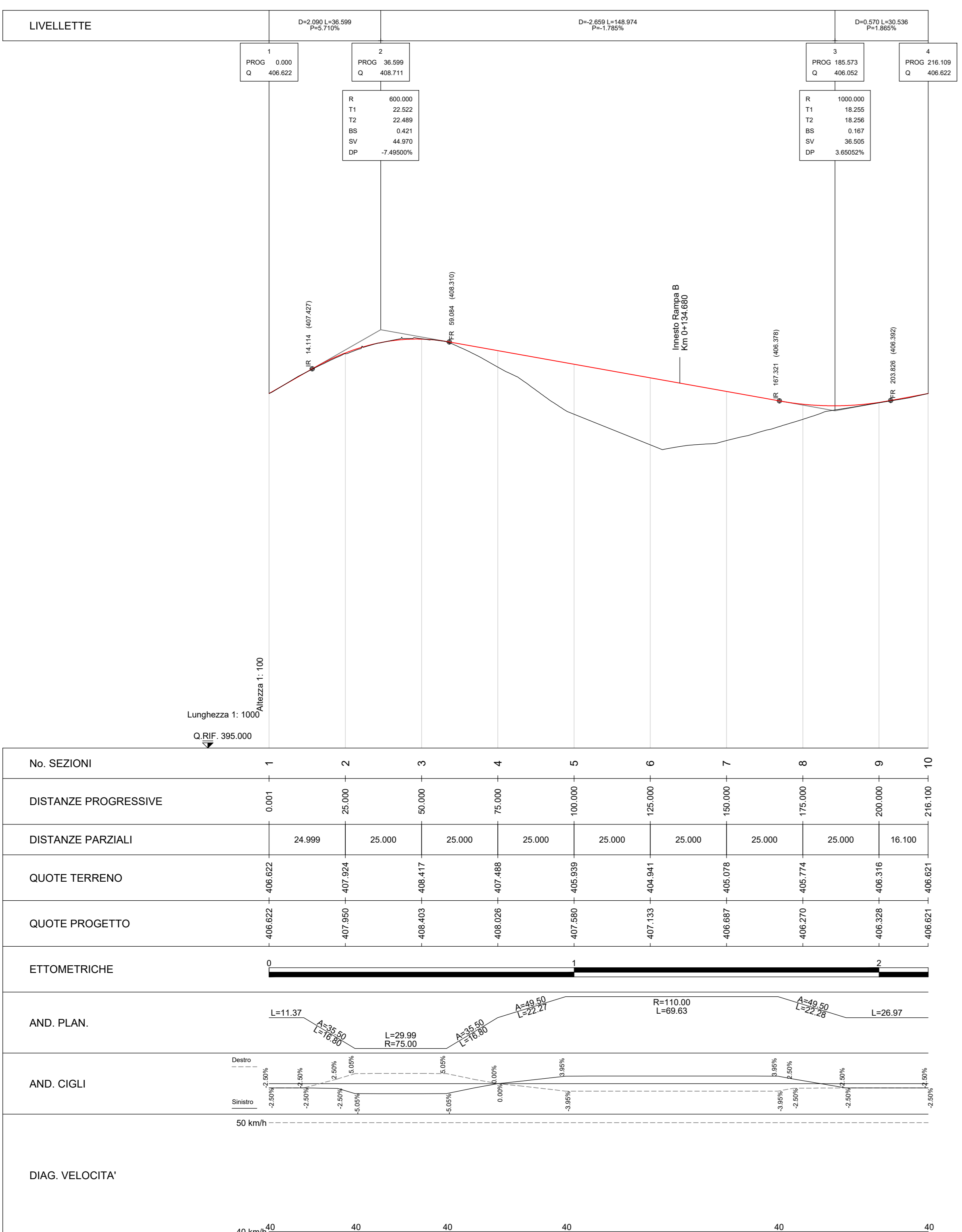
PROFILO DI PROGETTO ADEGUAMENTO VIABILITA' ESISTENTE - SCALA 1:1000/1:100
