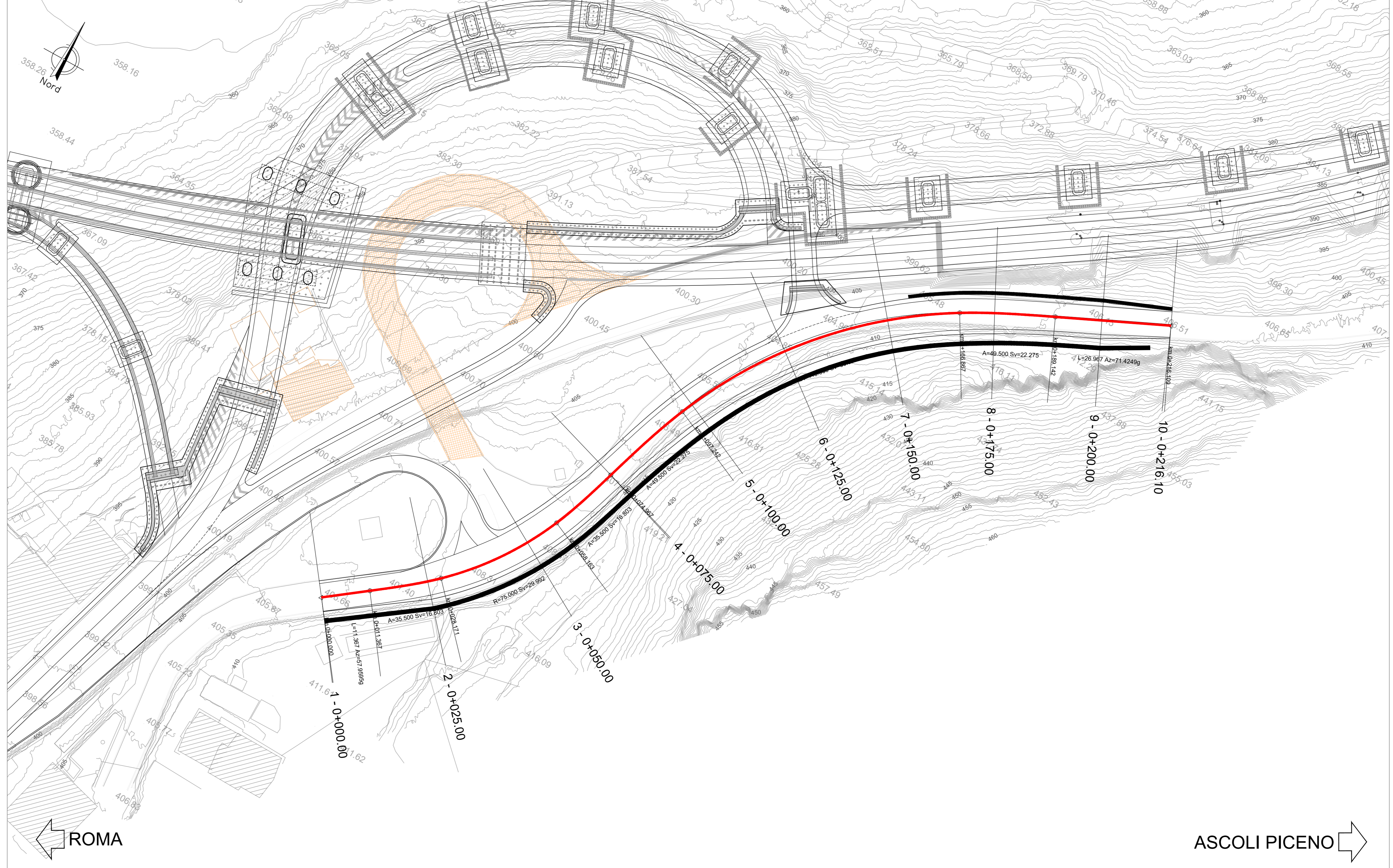
PLANIMETRIA DI PROGETTO E TRACCIAMENTO ADEGUAMENTO VIABILITA' ESISTENTE - SCALA 1:500
