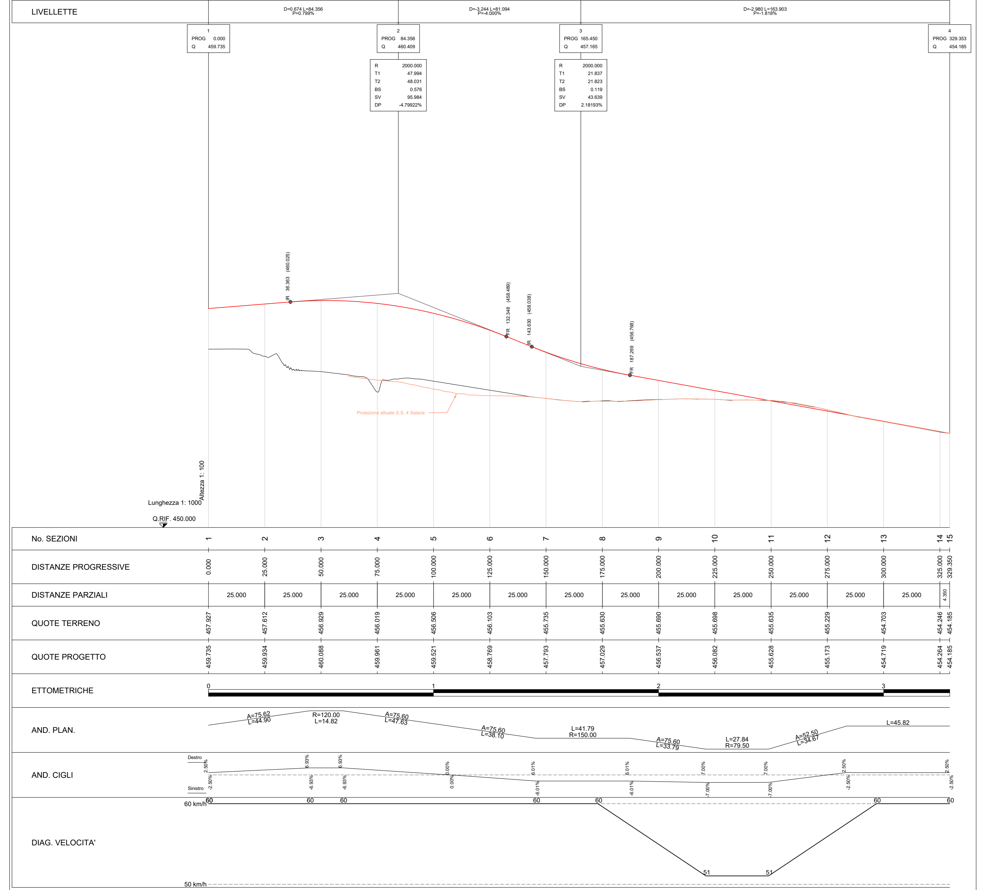
PROFILO DI PROGETTO RAMPA FAVALANCIATA - SCALA 1:1000/1:100
