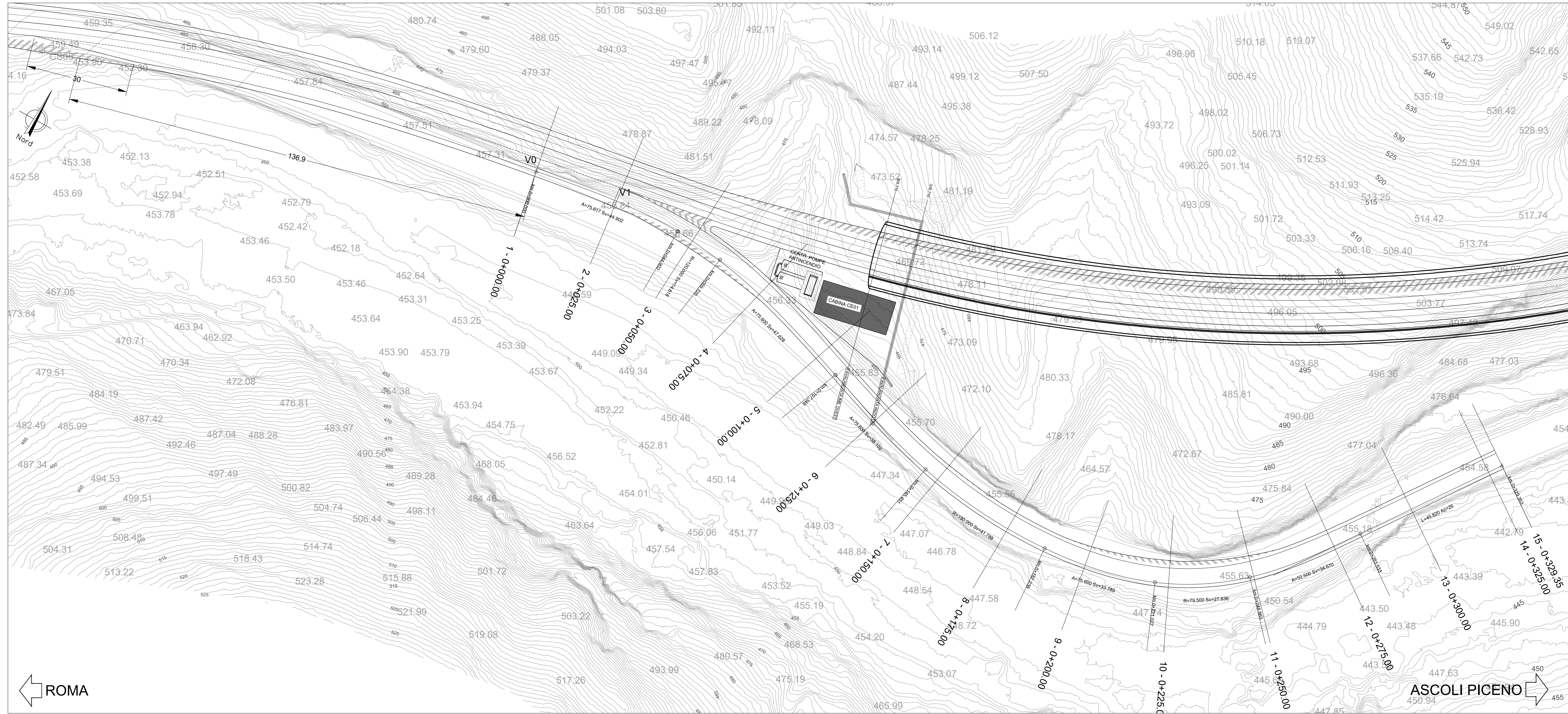
PLANIMETRIA DI PROGETTO E TRACCIAMENTO RAMPA FAVALANCIATA - SCALA 1:500
