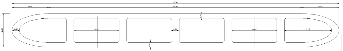
Figura -4: Pile tipo 4 – Sezione a 6 cellule
