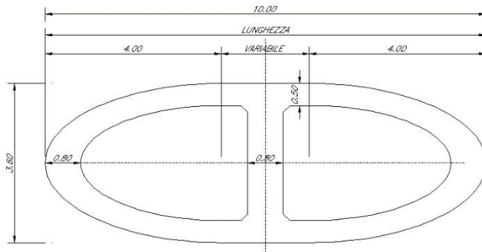
Figura -1: Pile tipo 1 – Sezione bicellulare
