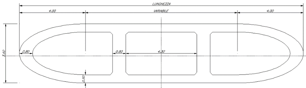
Figura -2: Pile tipo 2 – Sezione tricellulare
