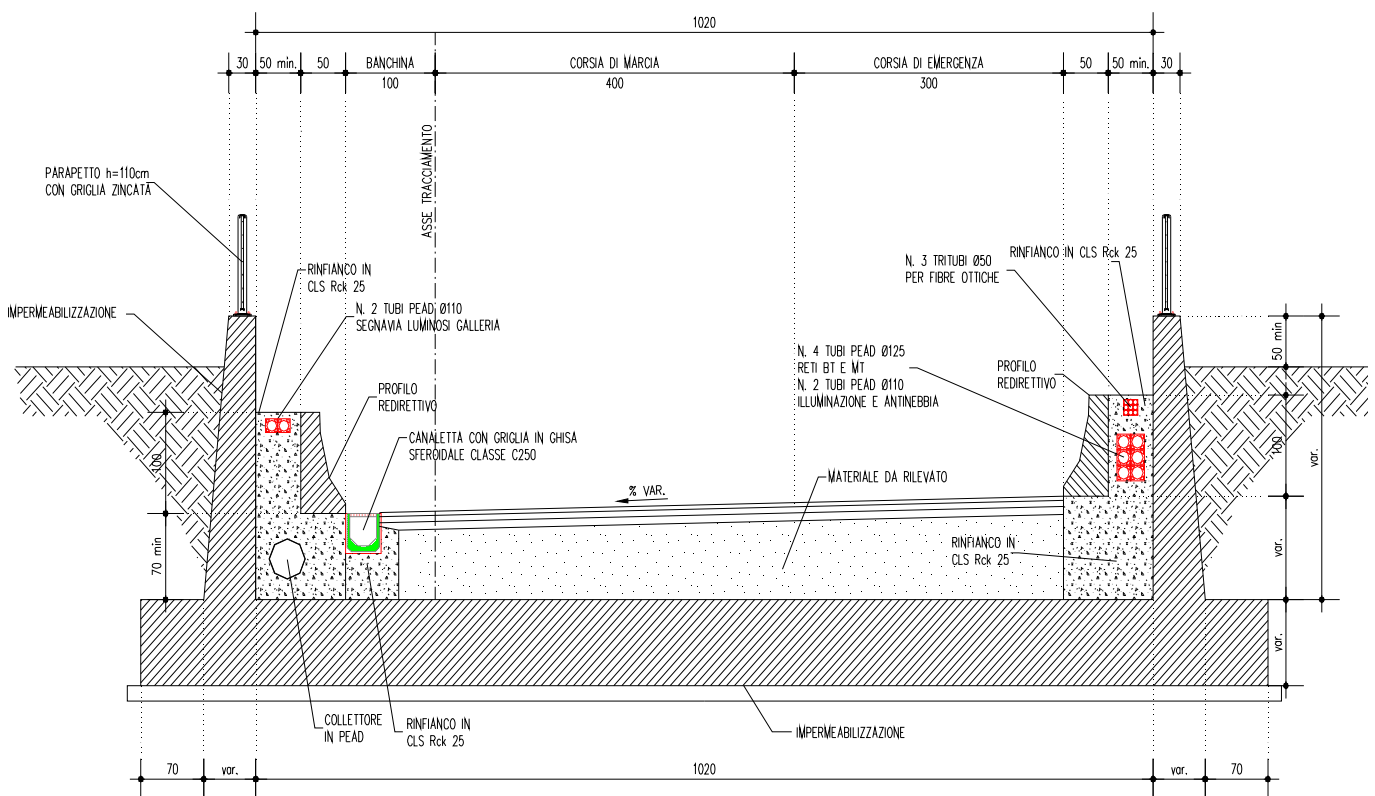
FIGURA 3.2.1 – SEZIONE TRASVERSALE TRINCEA DI MURI AD U
