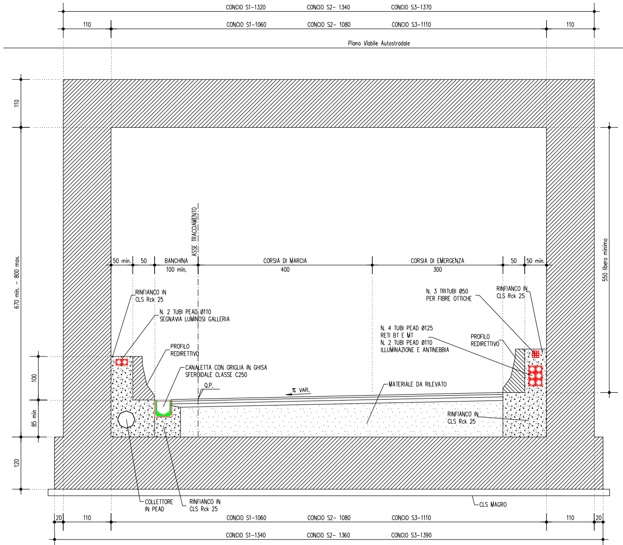
FIGURA 3.1.1 – SEZIONE TRASVERSALE SOTTOVIA SCATOLARE
