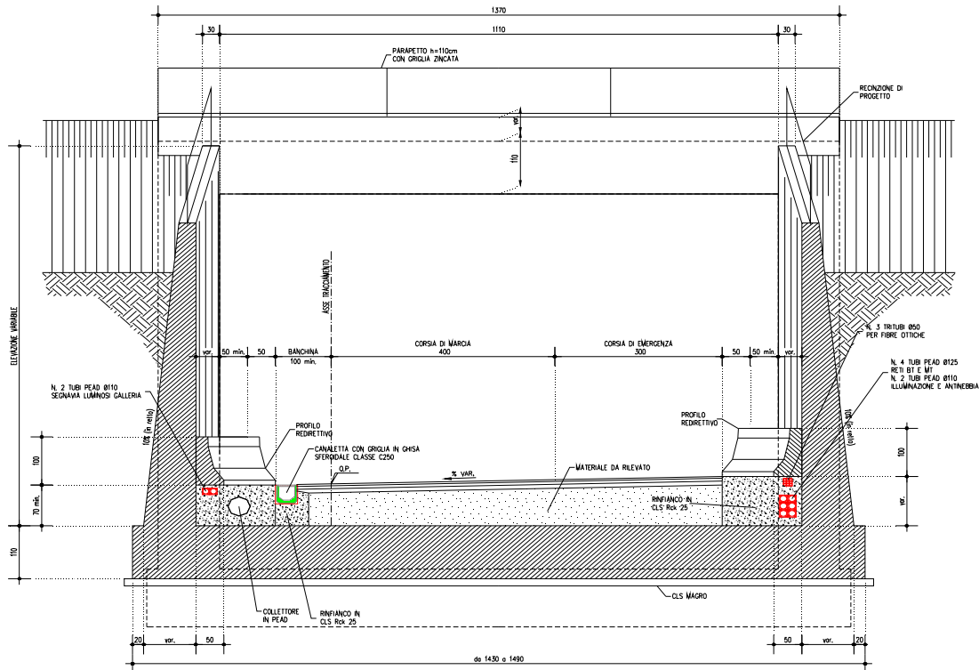
FIGURA 3.3.2 – SEZIONE TRASVERSALE MURO D'ALA AD U
