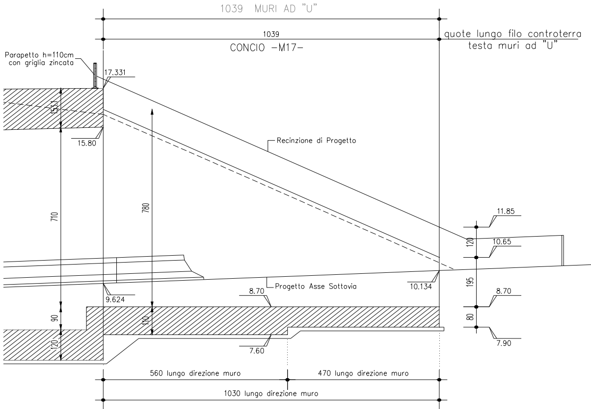
FIGURA 3.3.1 – SEZIONE LONGITUDINALE MURO D'ALA AD U
