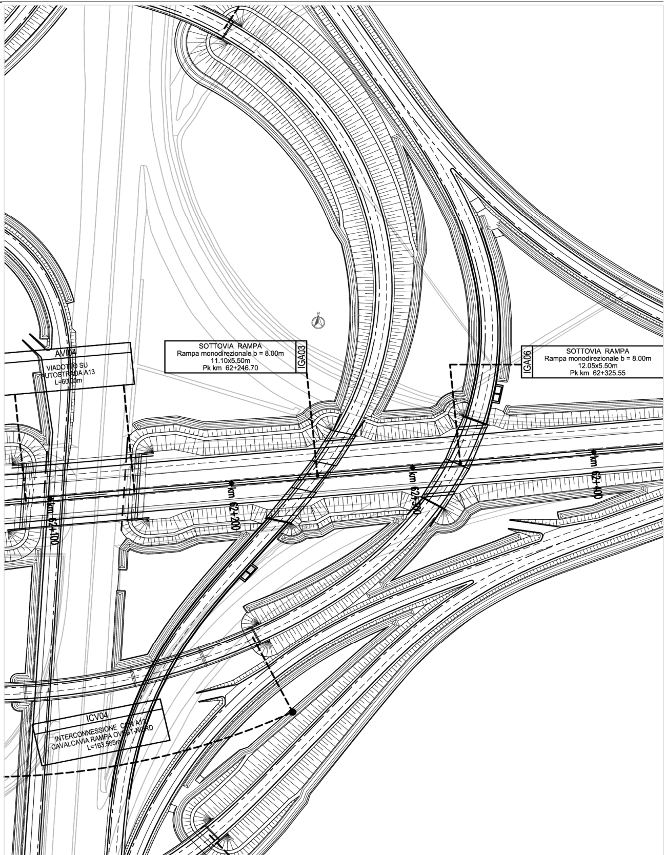
FIGURA 1.1 – SCHEMA PLANIMETRICO
