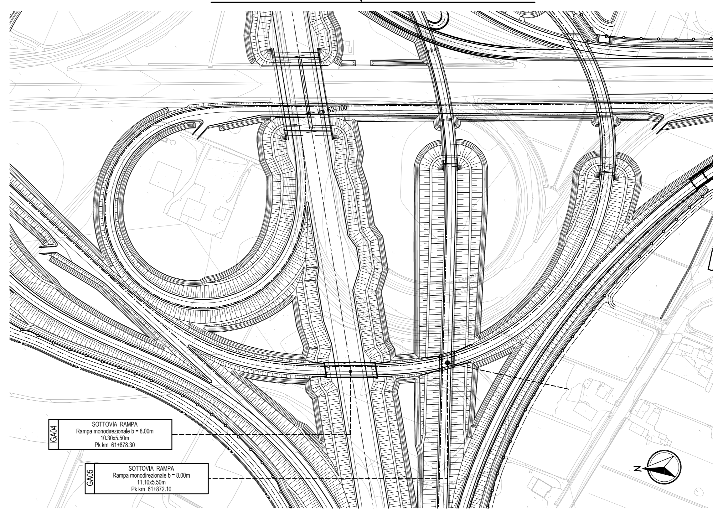
PLANIMETRIA DI INQUADRAMENTO 1:2000
