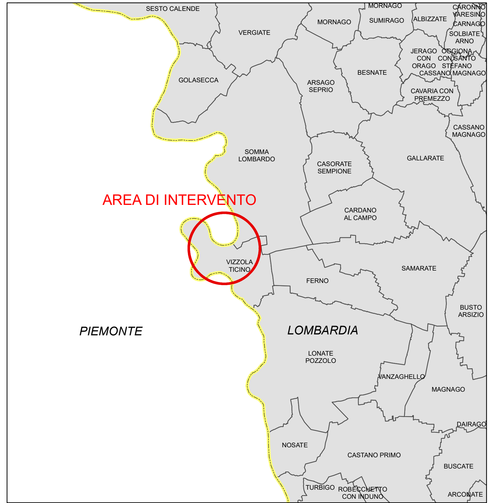
KEYPLAN - Scala 1:100.000
