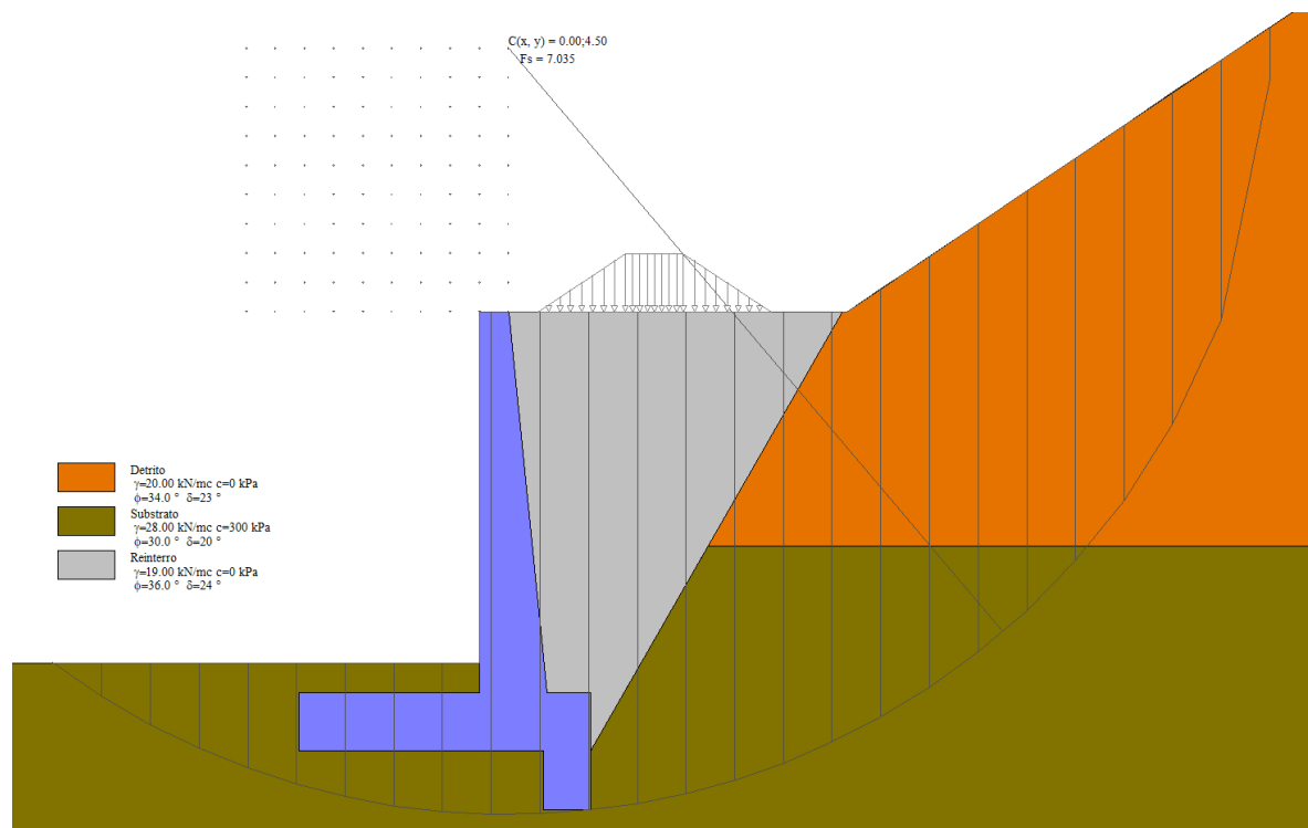
Figura n.11.4 – Superficie di rottura del terreno nella combinazione più critica
