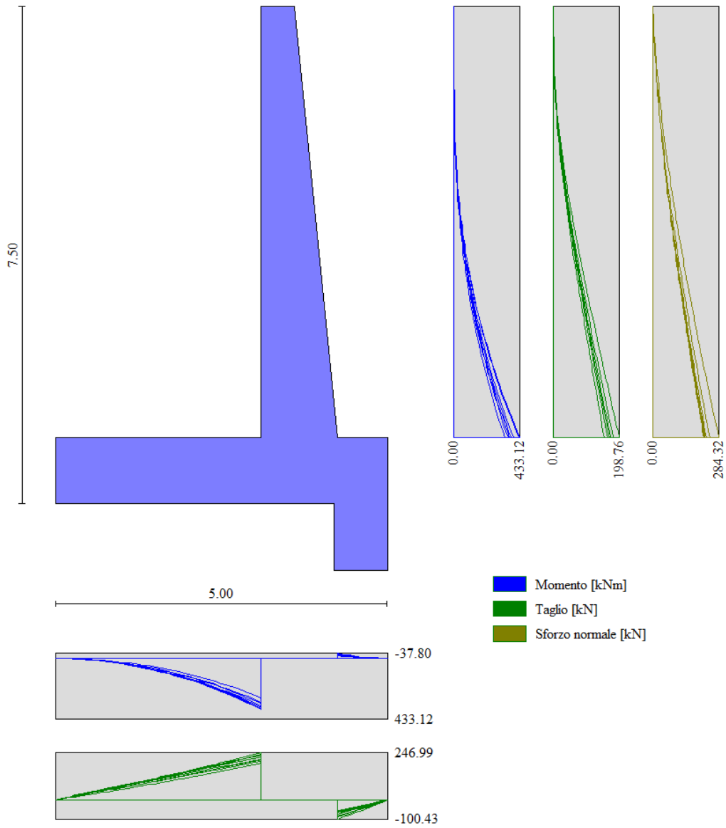
Figura n.11.3 – Involuppo delle sollecitazioni agenti
