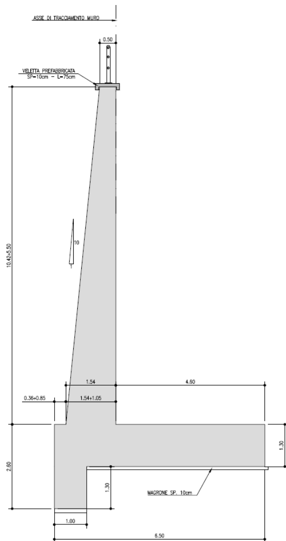
Figura n.1.1 – Geometria dell'opera – sezione tipo 1
