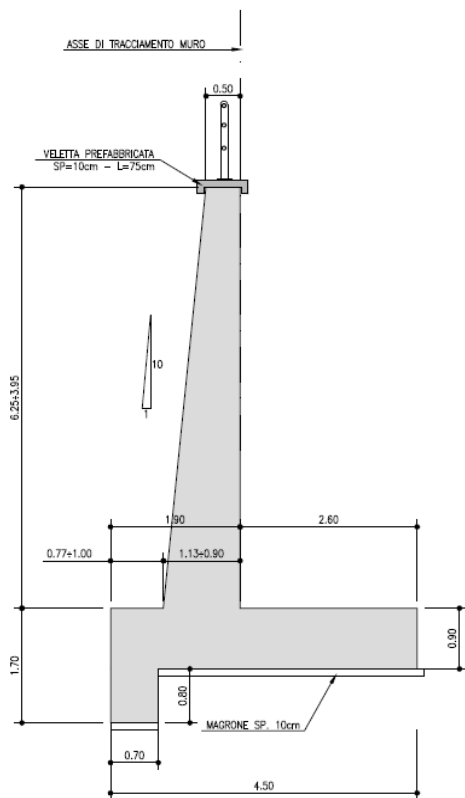
Figura n.1.1 – Geometria dell'opera – sezione tipo 2
