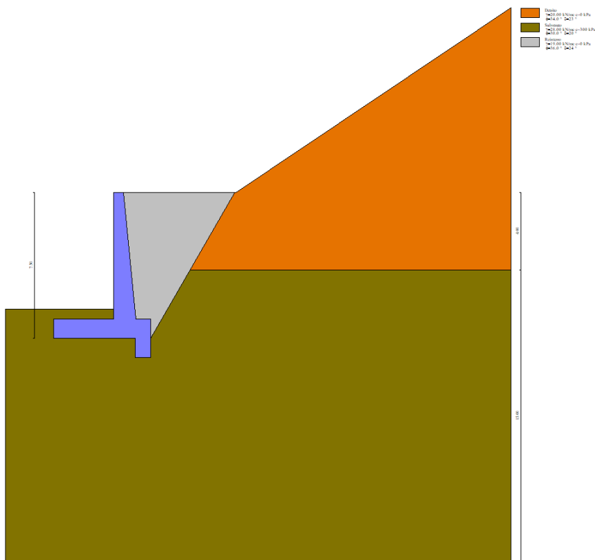
Figura n.11.2 – Sezione di verifica codice MAX15
