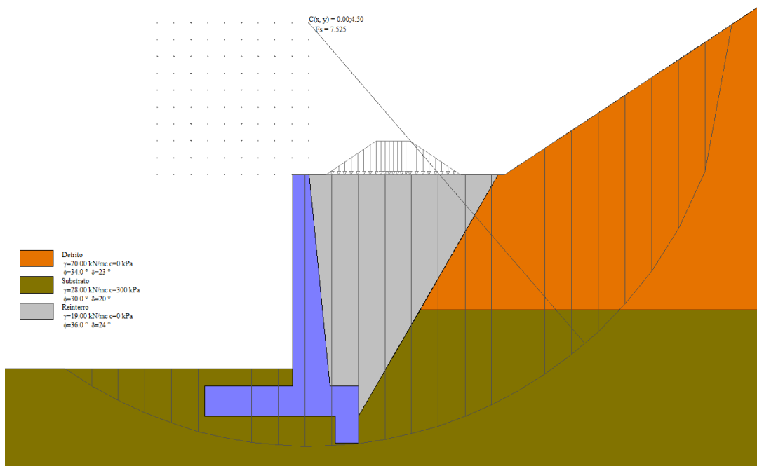
Figura n.10.4 – Superficie di rottura del terreno nella combinazione più critica
