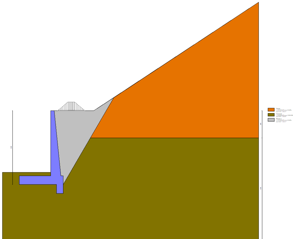
Figura n.9.2 – Sezione di verifica codice MAX15
