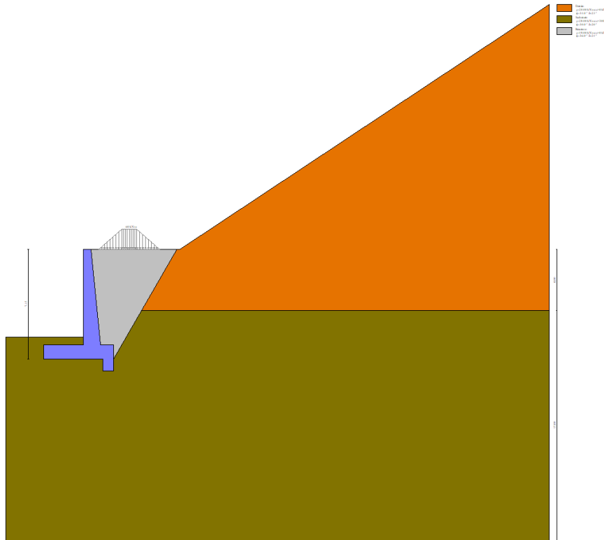
Figura n.10.2 – Sezione di verifica codice MAX15
