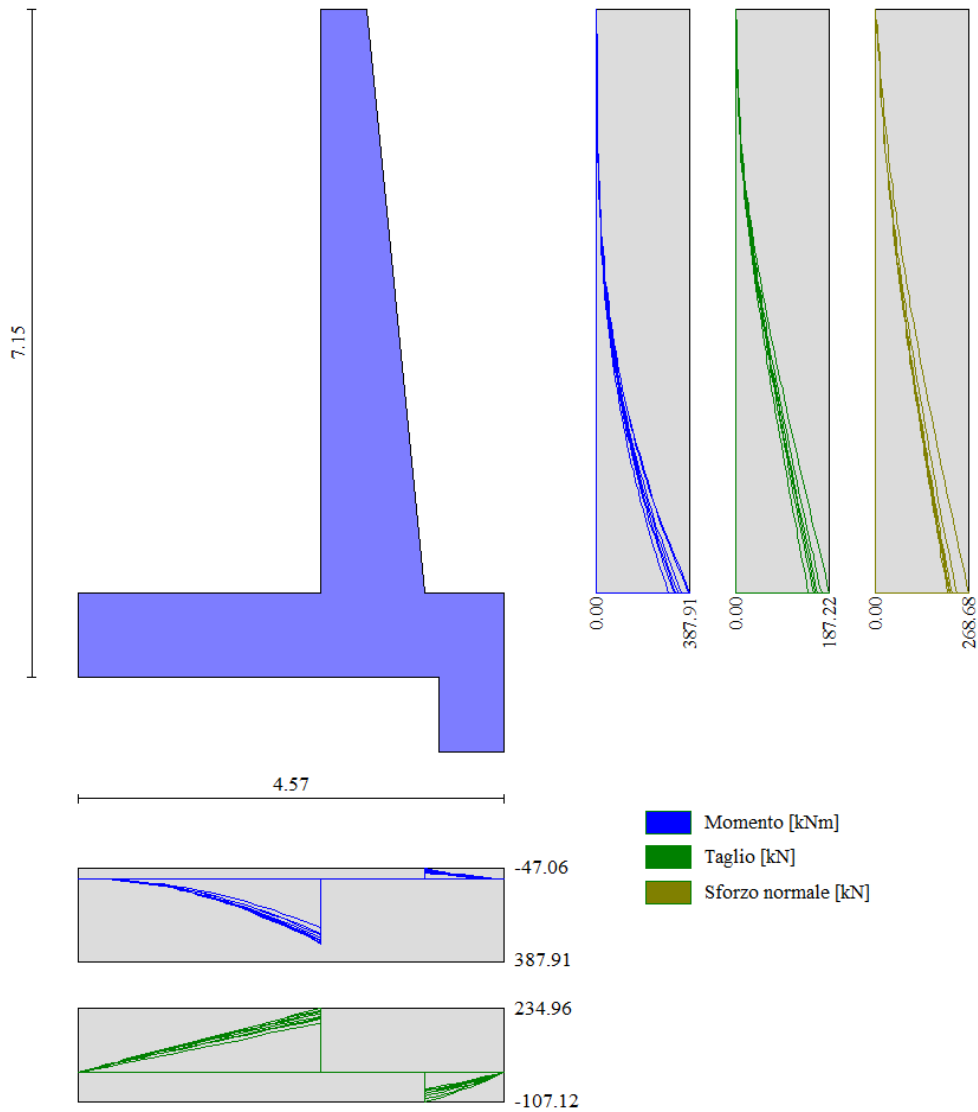
Figura n.10.3 – Involuppo delle sollecitazioni agenti
