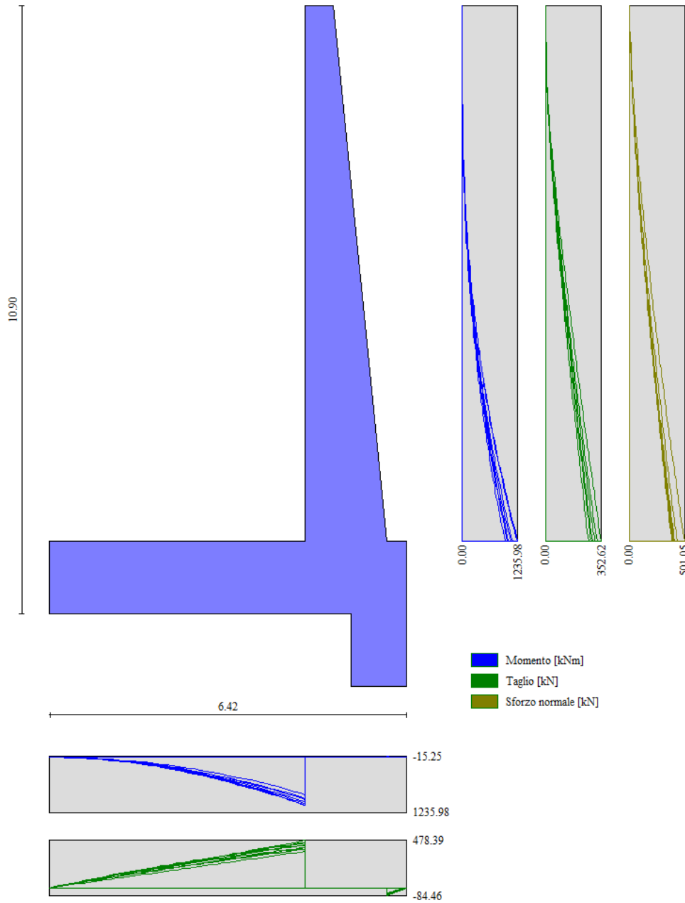
Figura n.9.3 – Inviluppo delle sollecitazioni agenti
