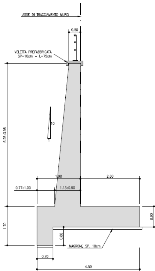
Figura n.10.1 – Carpenteria sezione tipo 2
