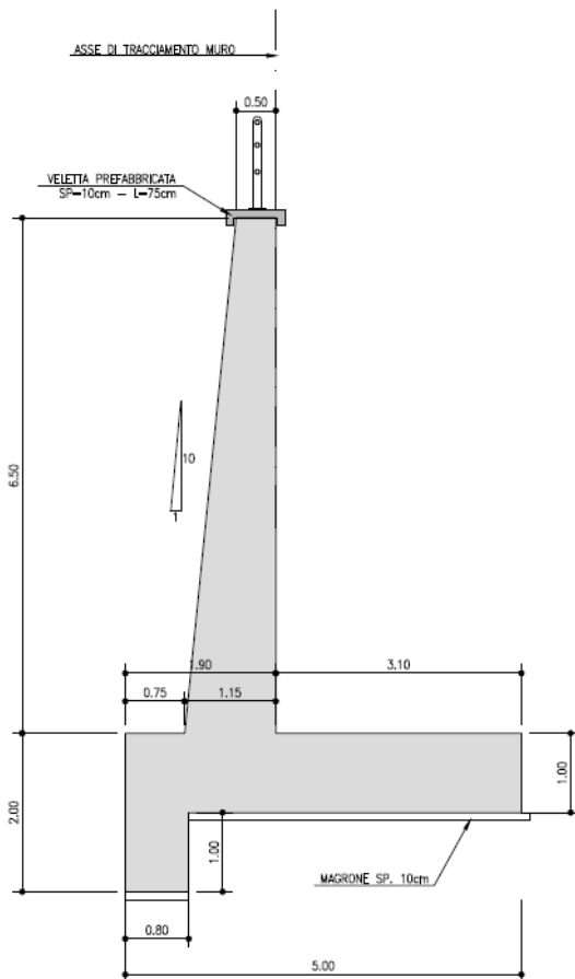
Figura n.11.1 – Carpenteria sezione tipo 3
