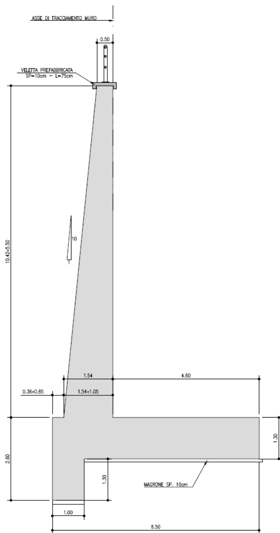
Figura n.9.1 – Carpenteria sezione tipo 1
