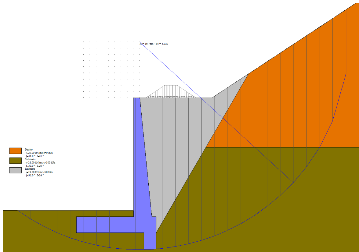
Figura n.9.4 – Superficie di rottura del terreno nella combinazione più critica
