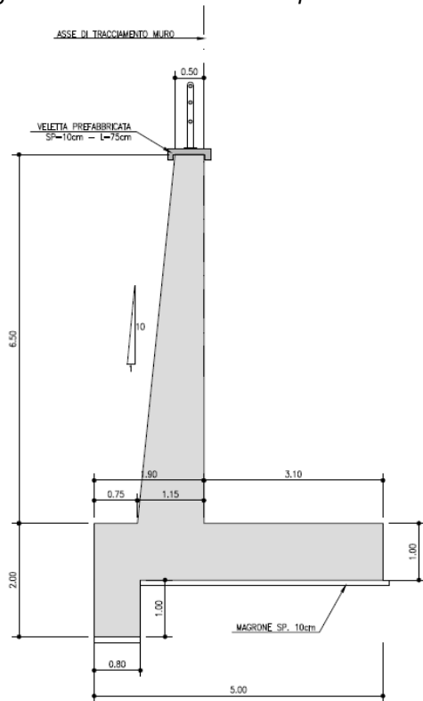
Figura n.1.3 – Geometria dell'opera – sezione tipo 3
