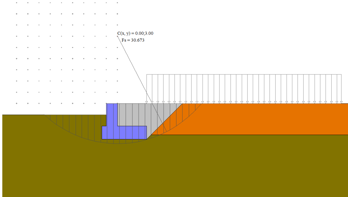
Figura n.11.4 – Superficie di rottura del terreno nella combinazione più critica
