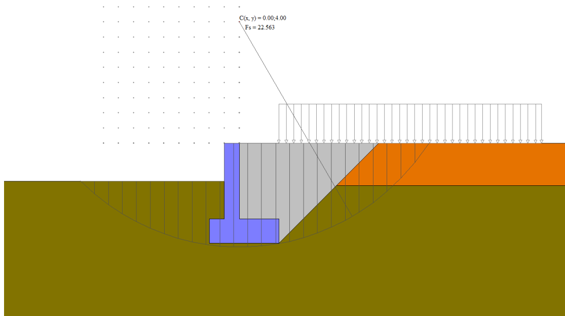
Figura n.10.4 – Superficie di rottura del terreno nella combinazione più critica
