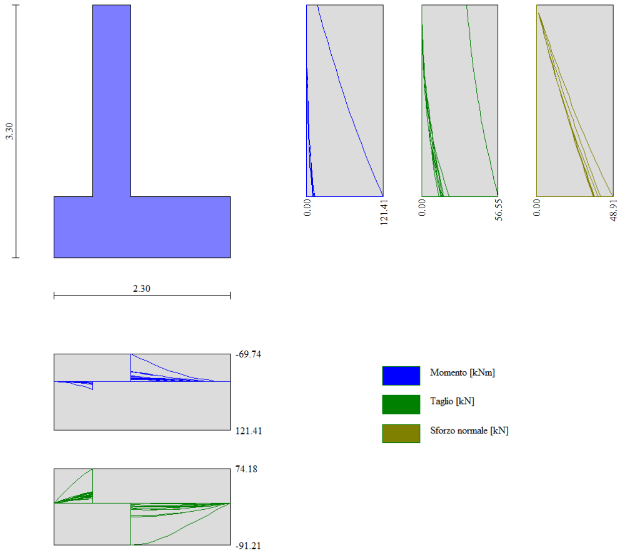
Figura n.10.3 – Involuppo delle sollecitazioni agenti
