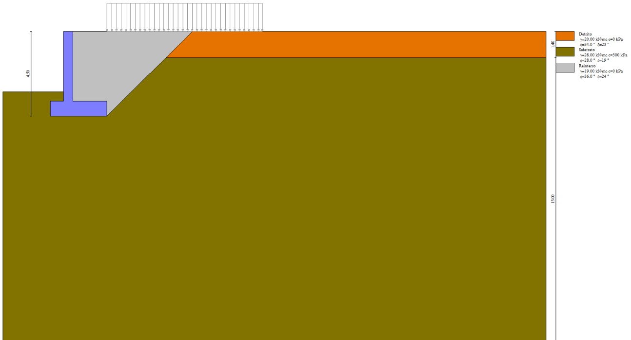
Figura n.9.2 – Sezione di verifica codice MAX15
