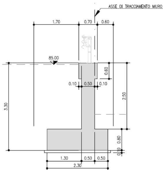
Figura n.1.2 – Geometria dell'opera – sezione tipo 2
