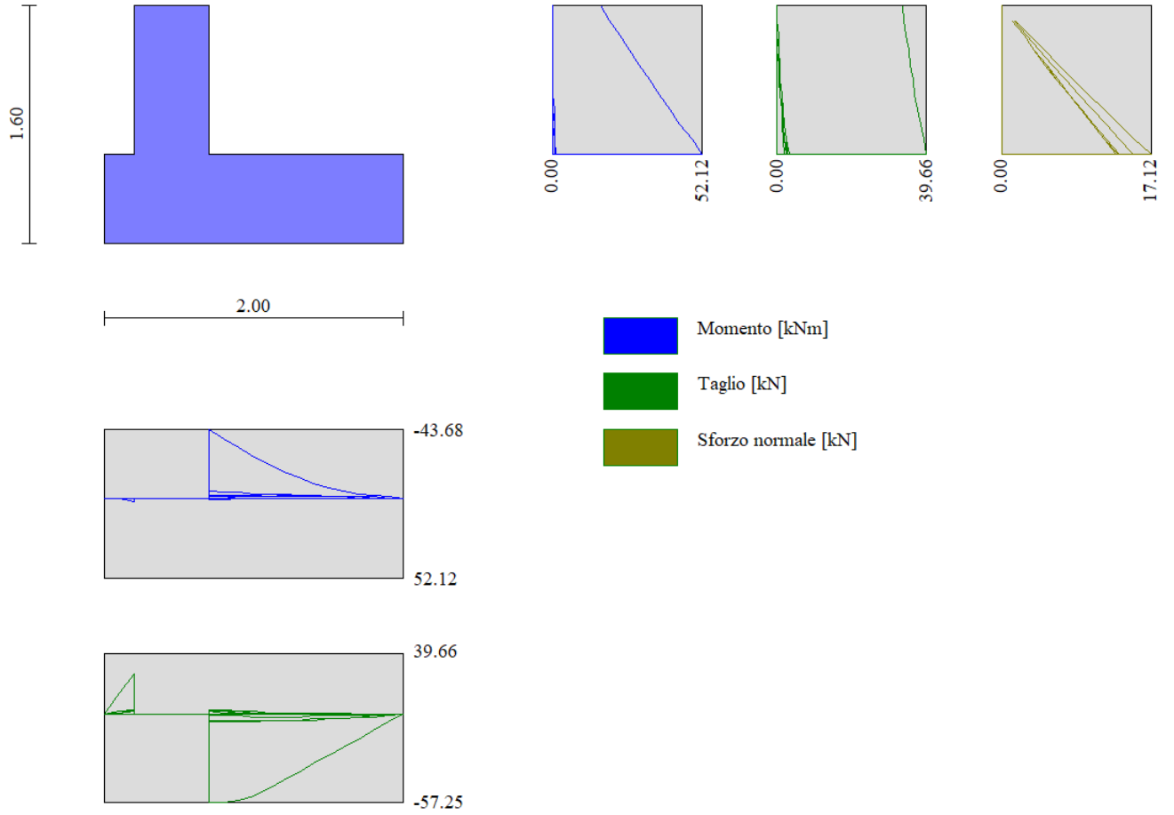
Figura n.11.3 – Involuppo delle sollecitazioni agenti
