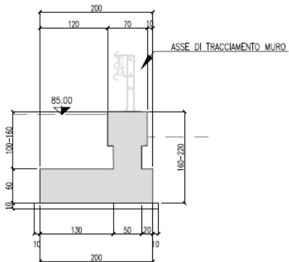
Figura n.11.1 – Carpenteria sezione tipo 3
