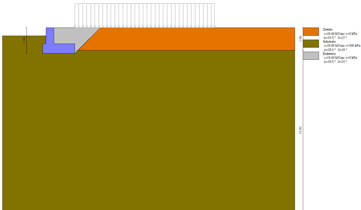
Figura n.11.2 – Sezione di verifica codice MAX15
