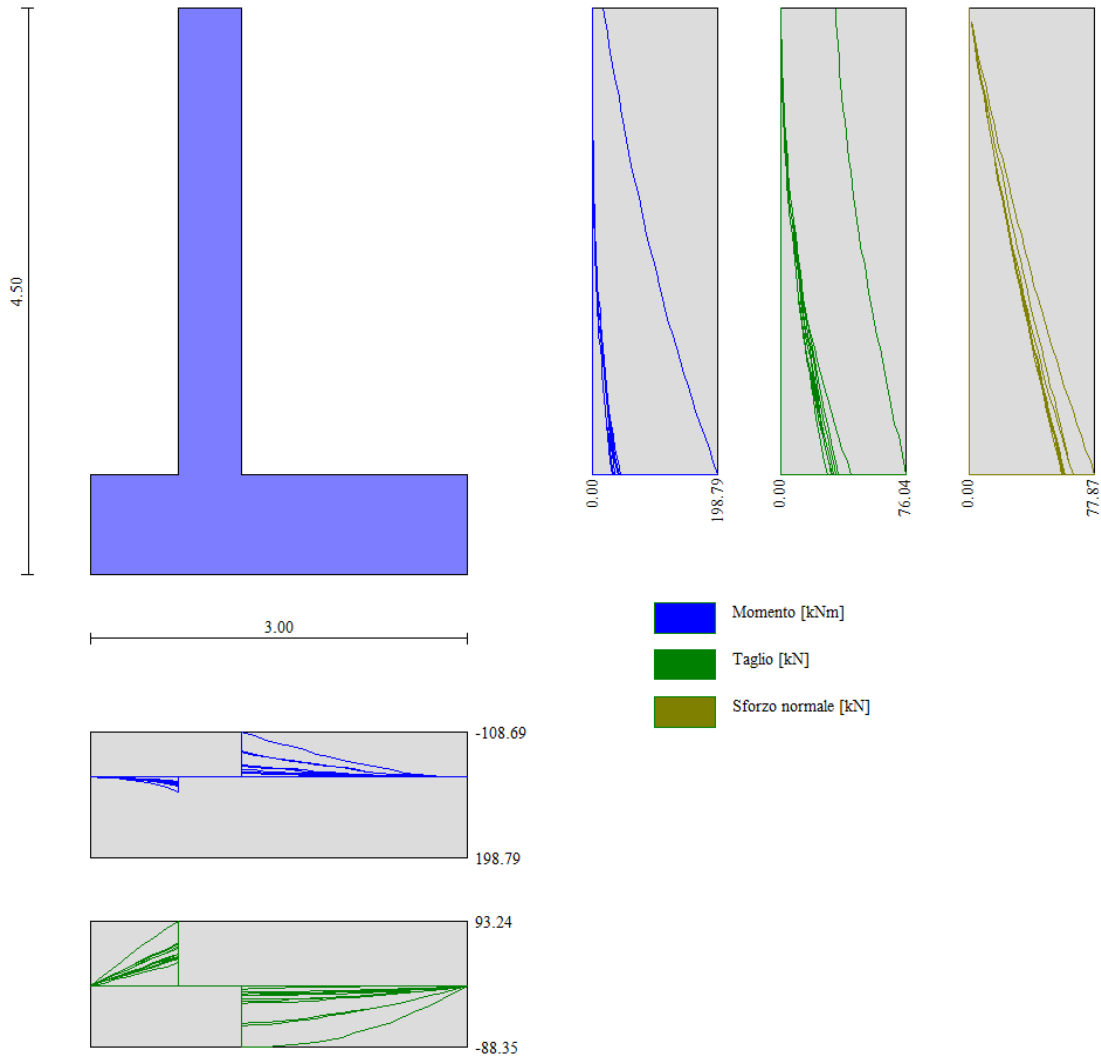
Figura n.9.3 – Involuppo delle sollecitazioni agenti
