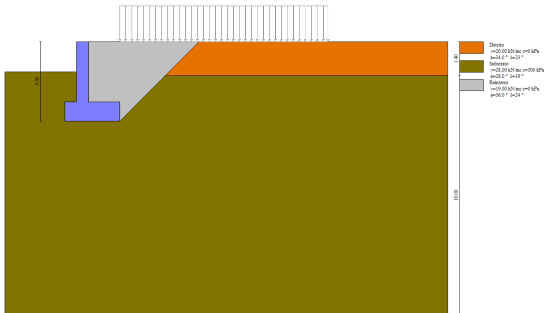
Figura n.10.2 – Sezione di verifica codice MAX15
