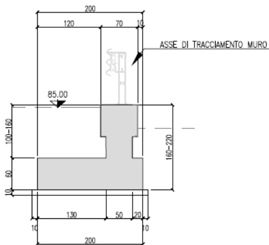
Figura n.1.3 – Geometria dell'opera – sezione tipo 3
