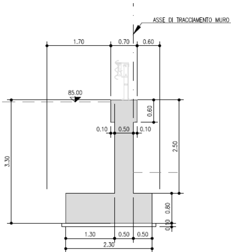
Figura n.10.1 – Carpenteria sezione tipo 2
