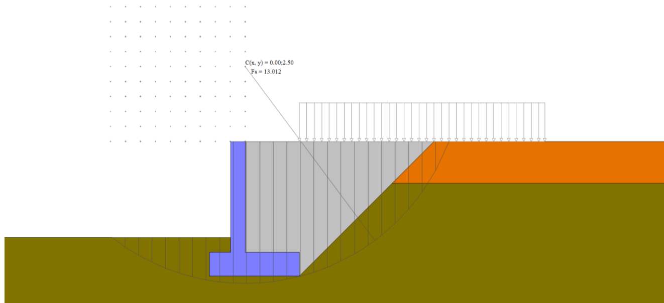
Figura n.9.4 – Superficie di rottura del terreno nella combinazione più critica
