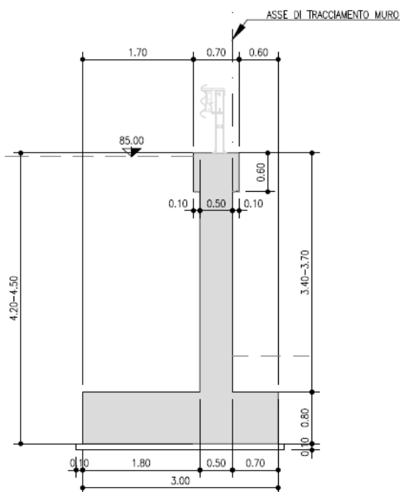
Figura n.1.1 – Geometria dell'opera – sezione tipo 1
