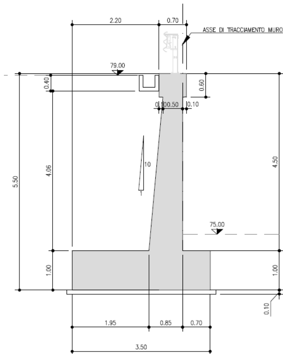
Figura n.1.1 – Geometria dell'opera – sezione tipo 1
