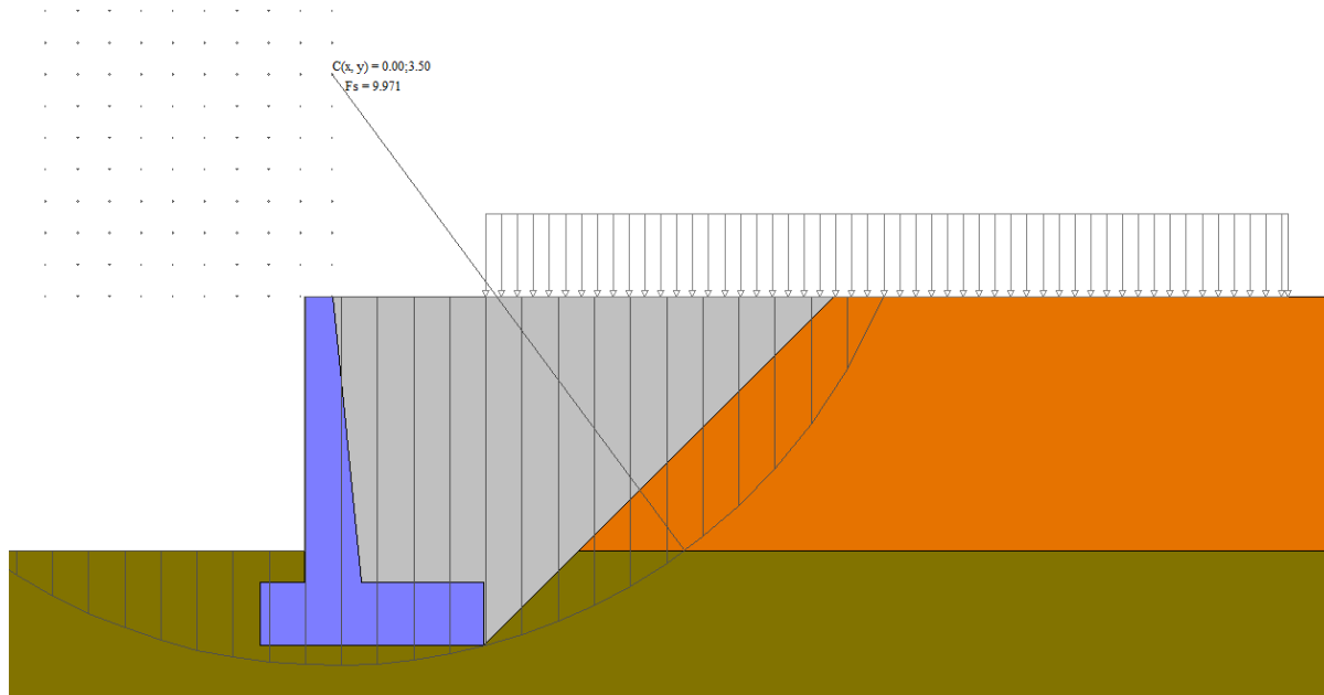
Figura n.10.4 – Superficie di rottura del terreno nella combinazione più critica
