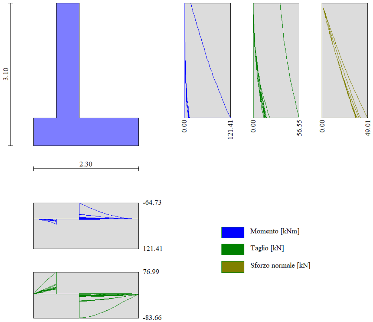
Figura n.10.3 – Involuppo delle sollecitazioni agenti
