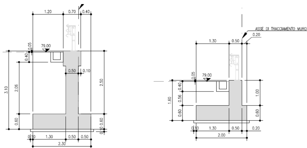
Figura n.1.2 – Geometria dell'opera – sezione tipo 2 ( a sinistra) e sezione tipo 3 ( a destra)
