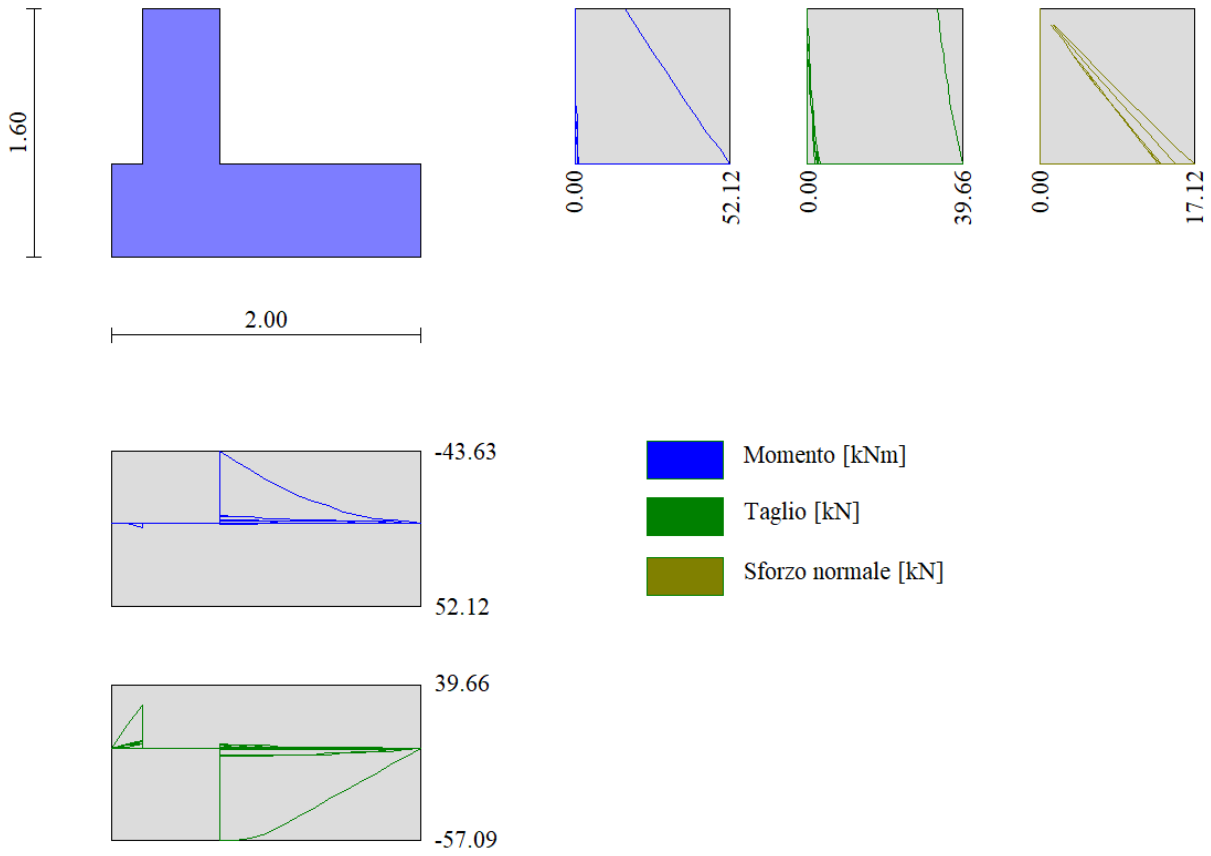
Figura n.11.3 – Involuppo delle sollecitazioni agenti
