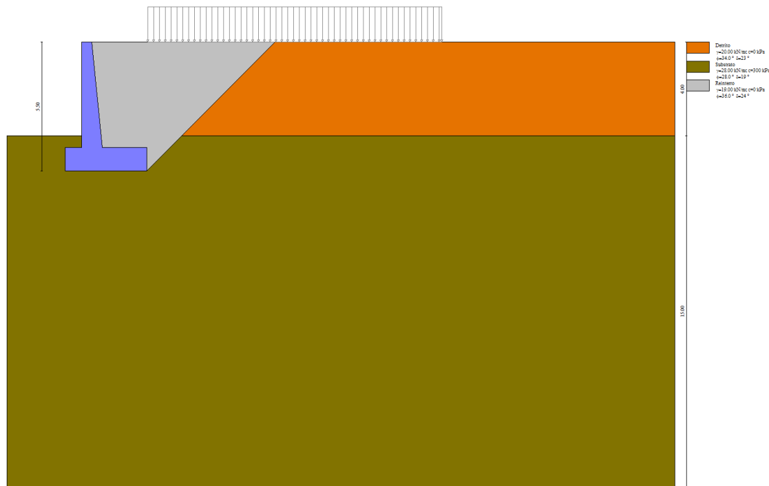
Figura n.10.2 – Sezione di verifica codice MAX15
