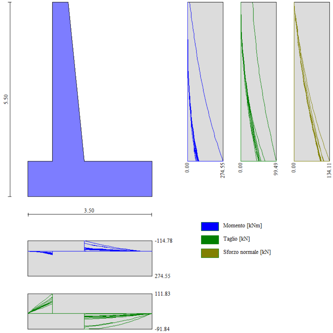
Figura n.10.3 – Involuppo delle sollecitazioni agenti
