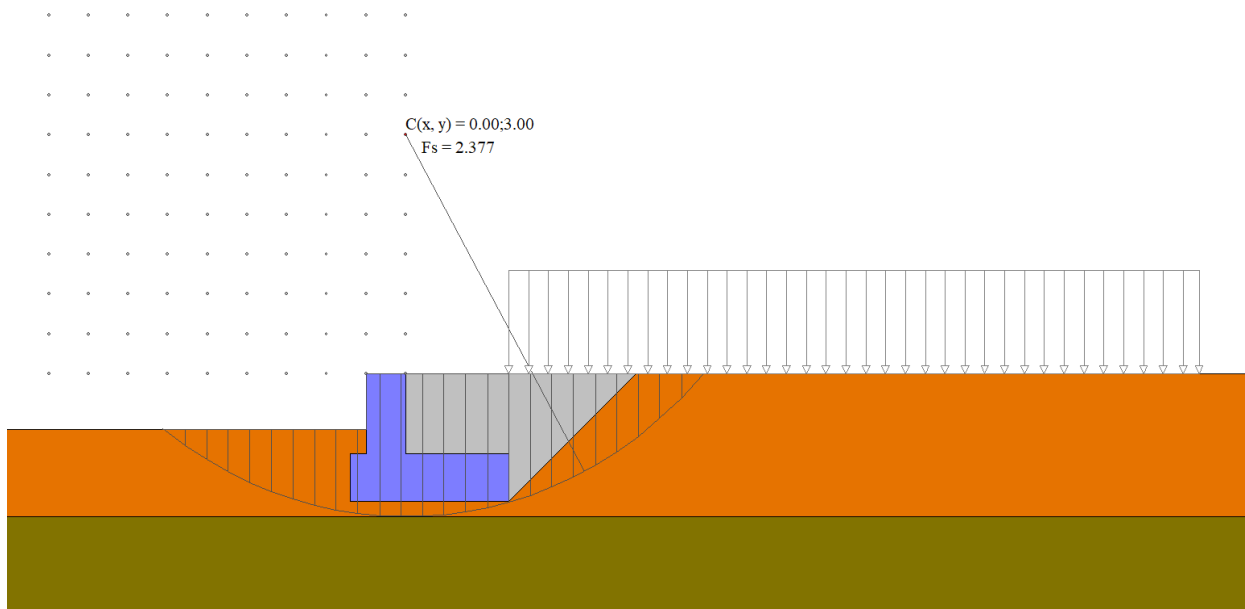
Figura n.11.4 – Superficie di rottura del terreno nella combinazione più critica
