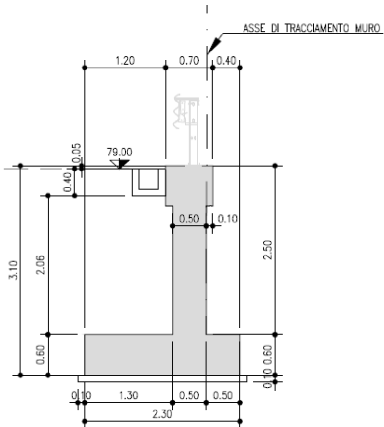
Figura n. 10.1 – Carpenteria sezione tipo 2
