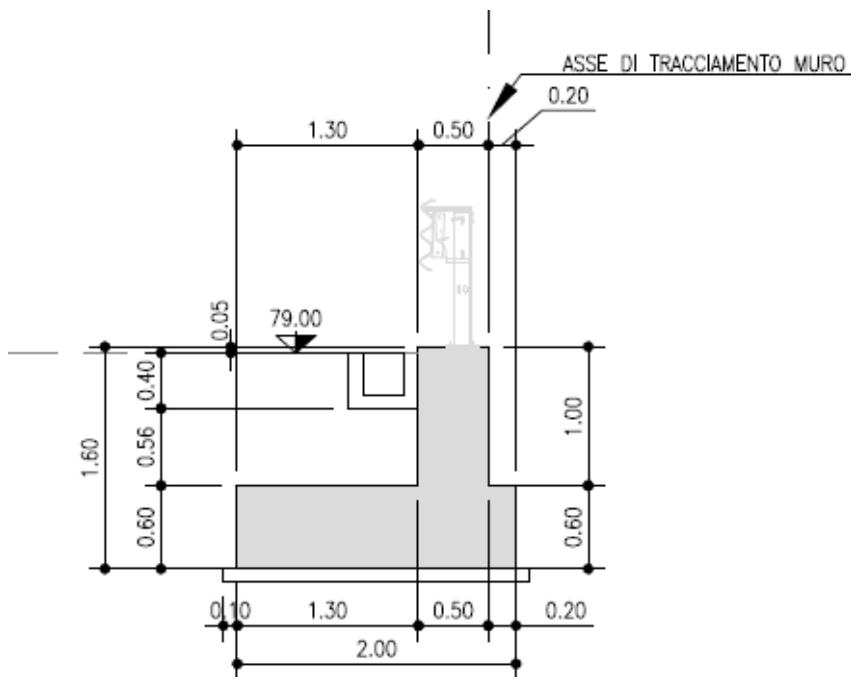
Figura n.11.1 – Carpenteria sezione tipo 3
