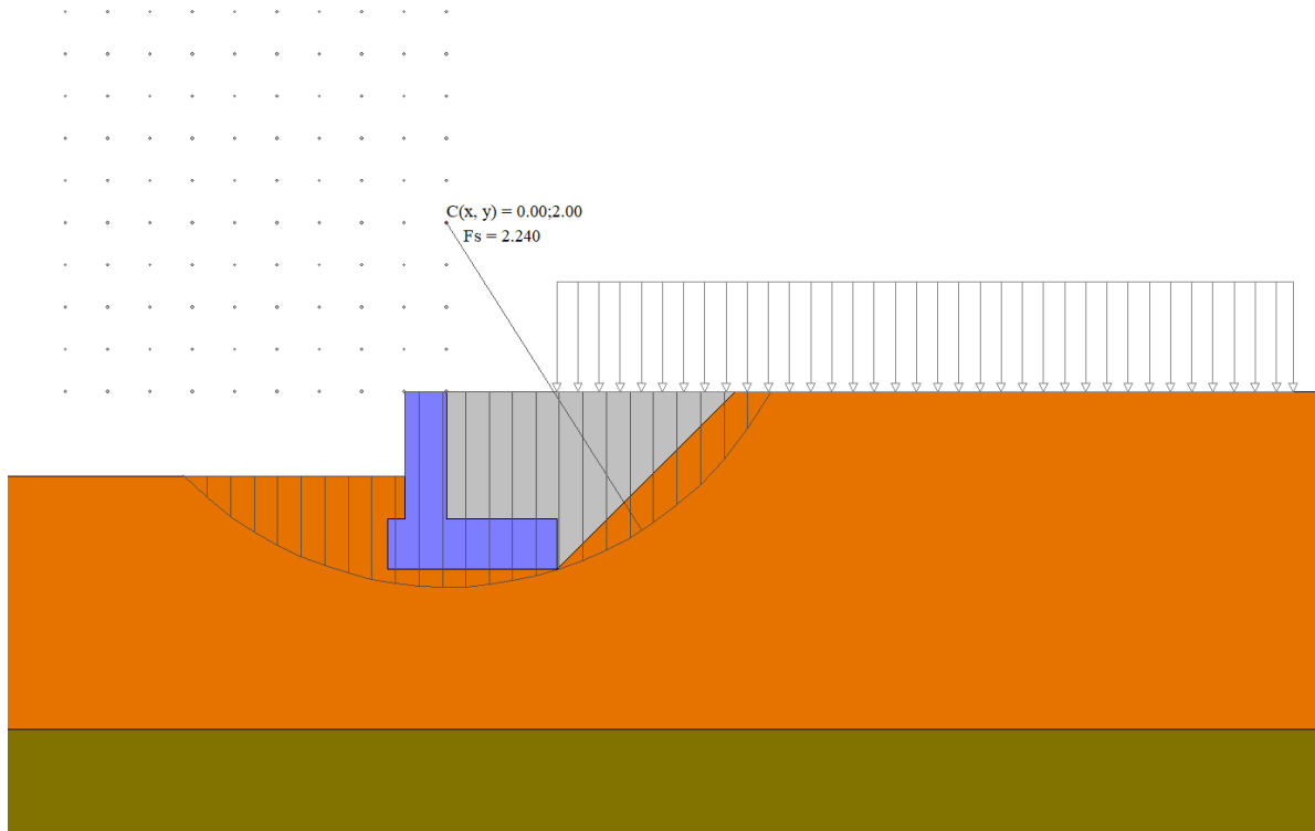
Figura n.10.4 – Superficie di rottura del terreno nella combinazione più critica
