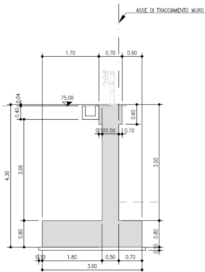
Figura n.9.1 – Carpenteria sezione tipo 1
