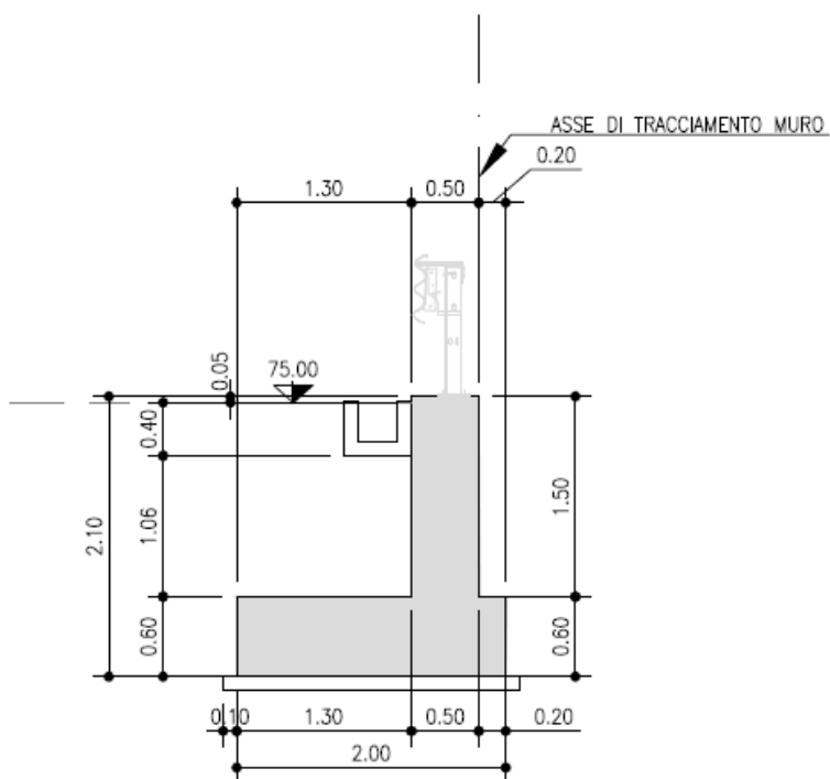
Figura n.10.1 – Carpenteria sezione tipo 2
