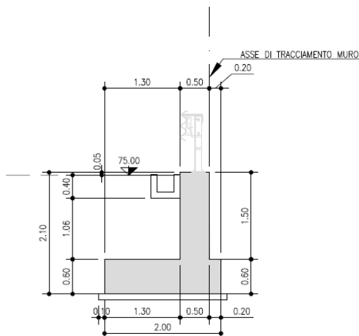
Figura n.1.2 – Geometria dell'opera – sezione tipo 2
