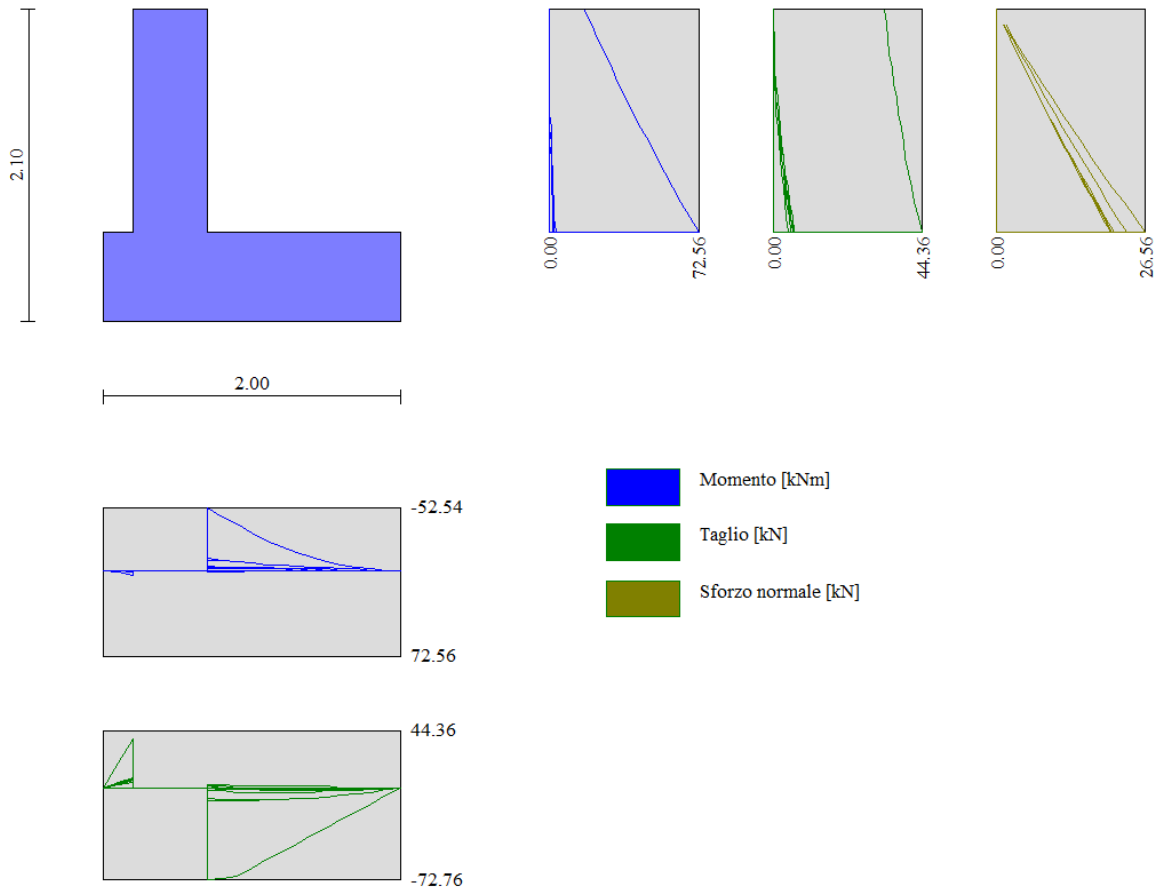
Figura n.10.3 – Involuppo delle sollecitazioni agenti
