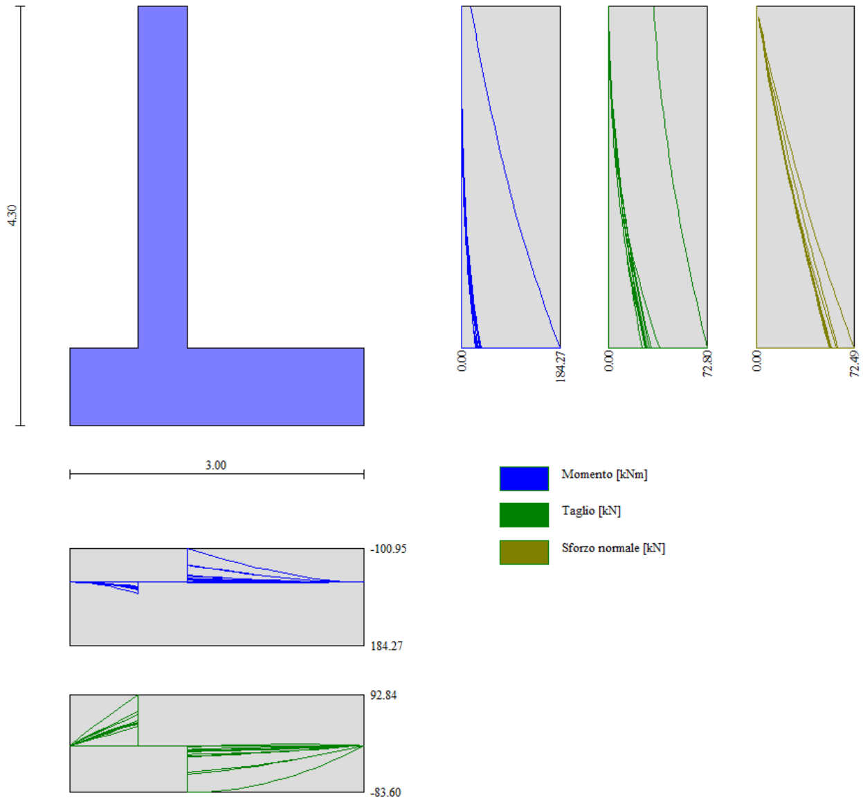
Figura n.9.3 – Inviluppo delle sollecitazioni agenti
