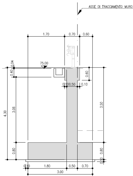
Figura n.1.1 – Geometria dell'opera – sezione tipo 1
