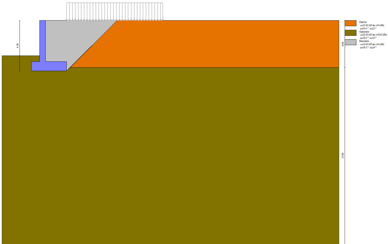
Figura n.9.2 – Sezione di verifica codice MAX15
