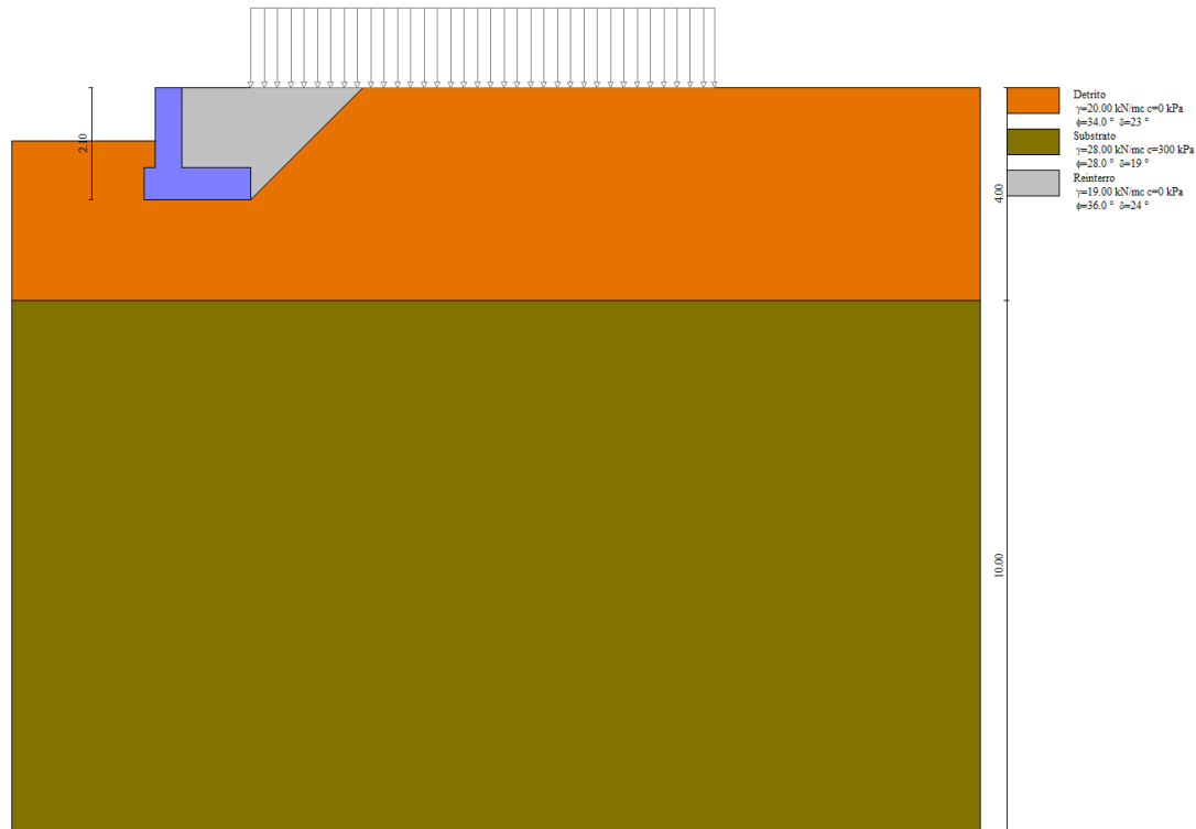
Figura n.10.2 – Sezione di verifica codice MAX15
