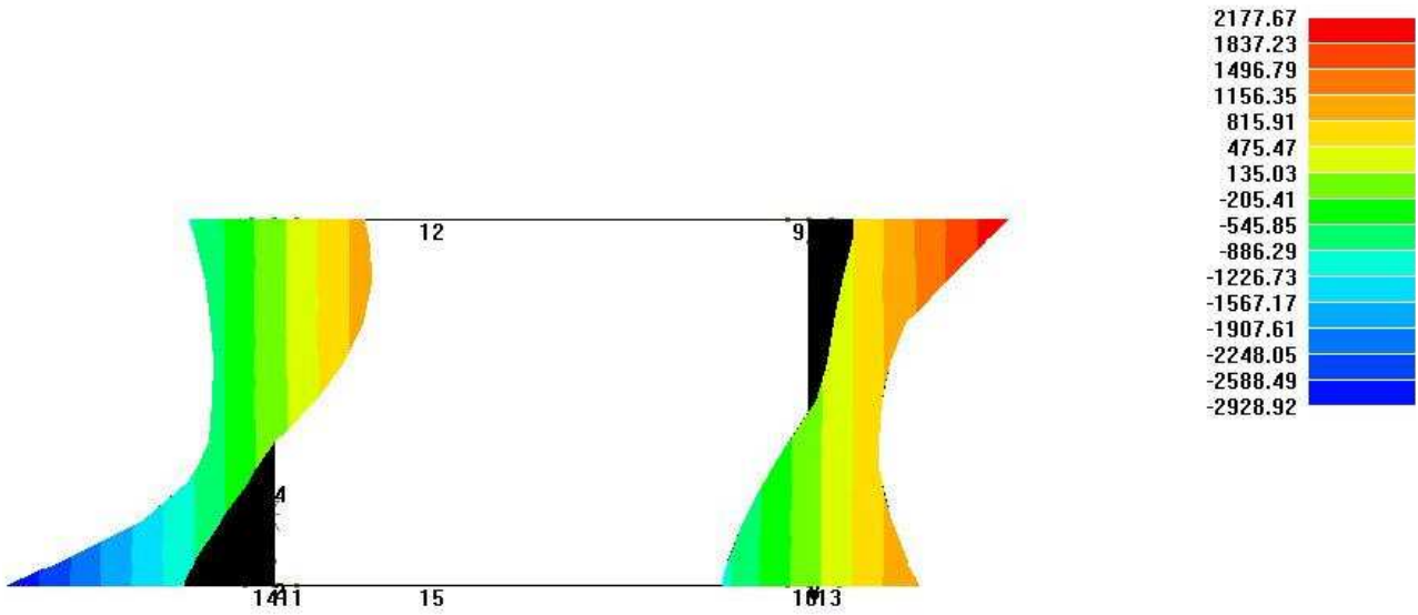
PROGETTO Inviluppo sollecitazioni Momento 3-3 [kN m]
