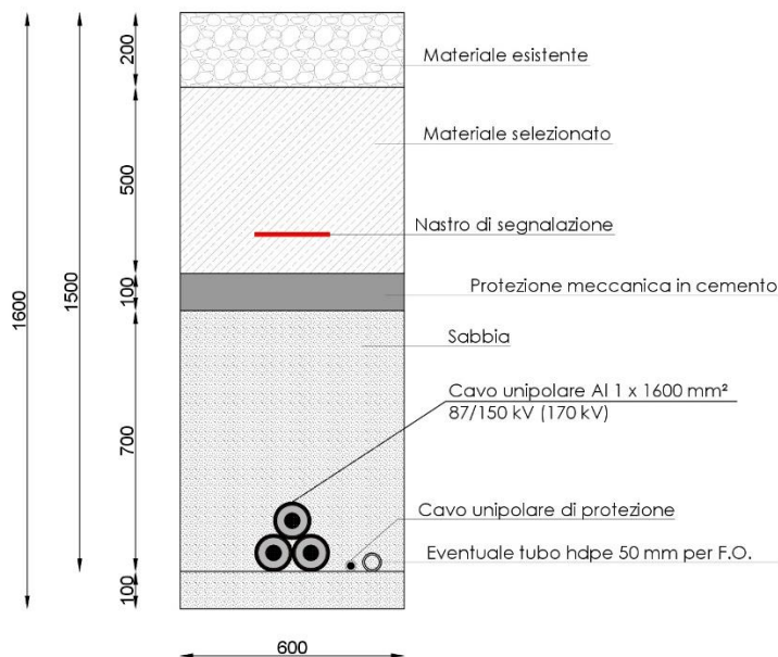
Figura 1 - Tipologico scavo per cavo AT
