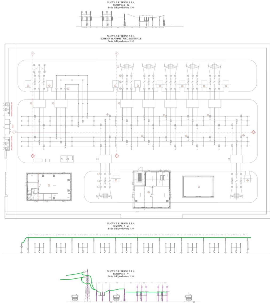
Figura 3.4: Nuova S.E. Terna S.p.A.
