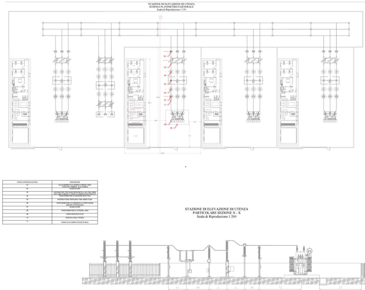
Figura 3.3: Nuova S.E.U. (Stazione di Elevazione di Utenza)
