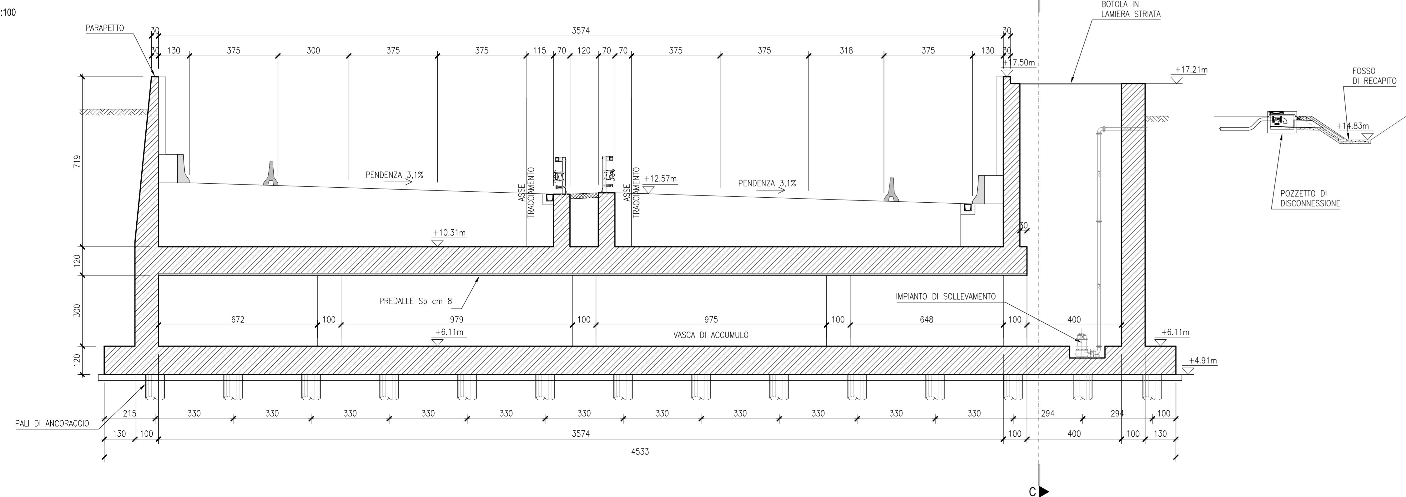
SEZIONE A-A CARPENTERIA SCALA 1:100
