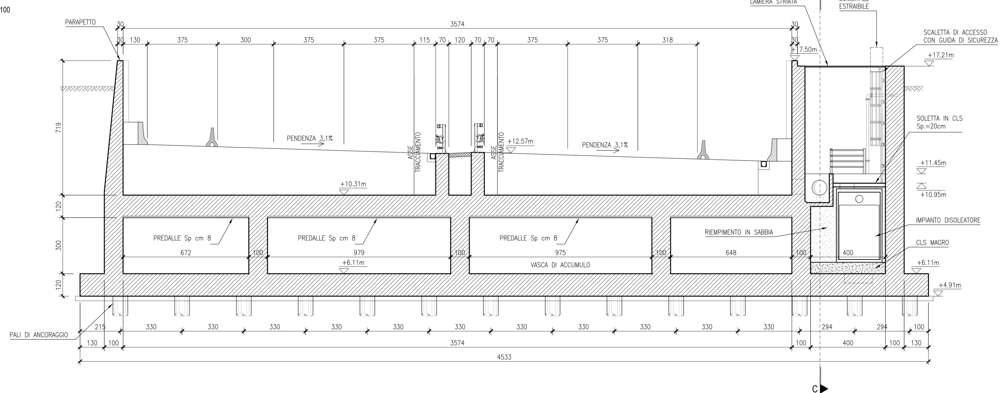
SEZIONE B-B CARPENTERIA SCALA 1:100
