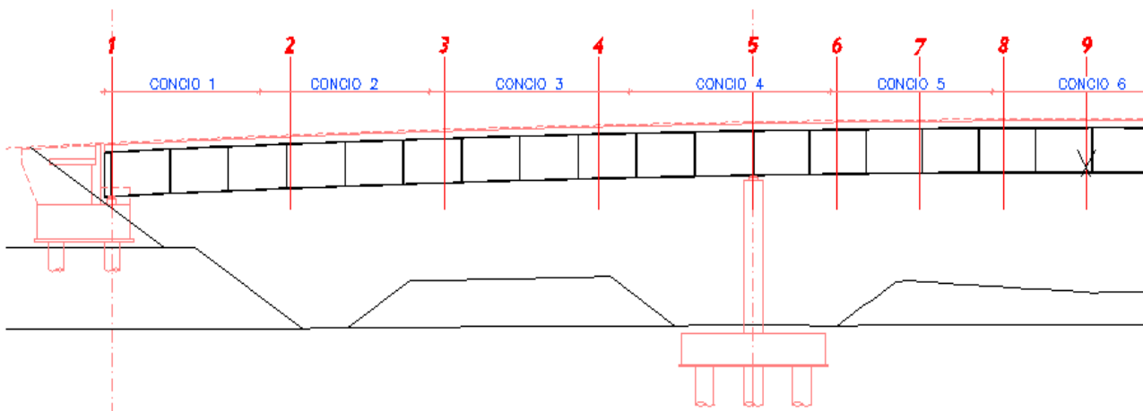
FIGURA 28 SUDDIVISIONE DELLE TRAVI IN CONCI
