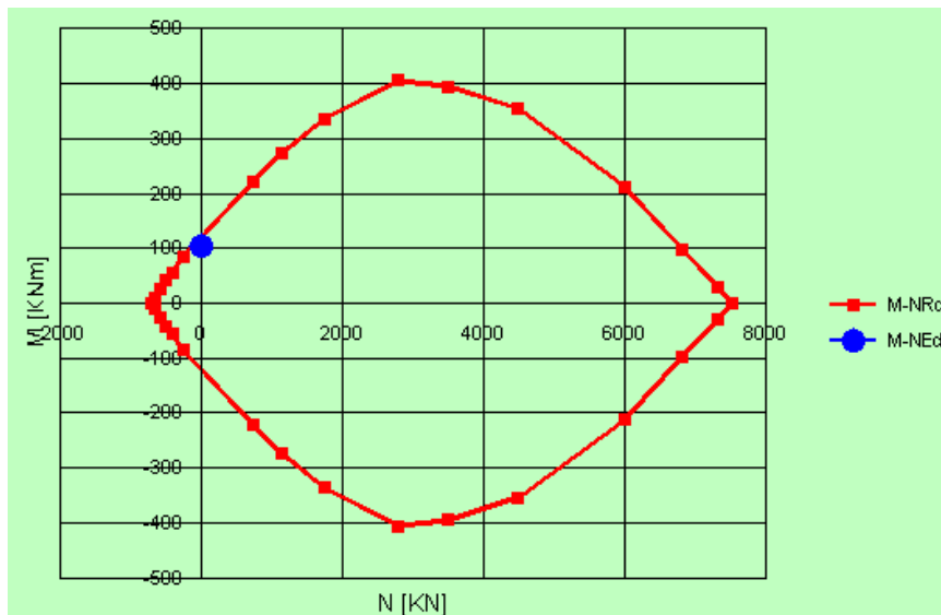
FIGURA 27 DOMINIO RESISTENTE SEZIONE LONGITUDINALE CAMAPATA SOLETTA
