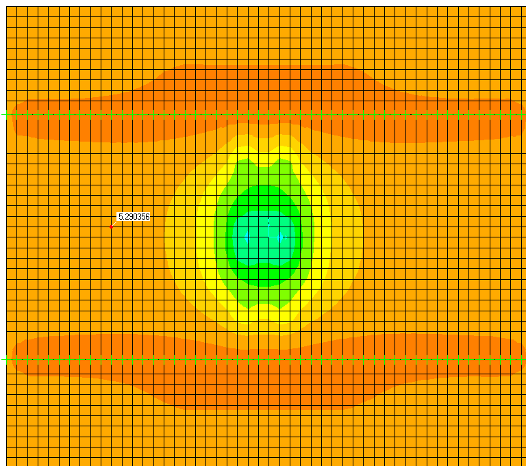
FIGURA 18 MOMENTO FLETTENTE - SOLLECITA LE FIBRE PARALLELE ALLE TRAVI PRINCIPALI
