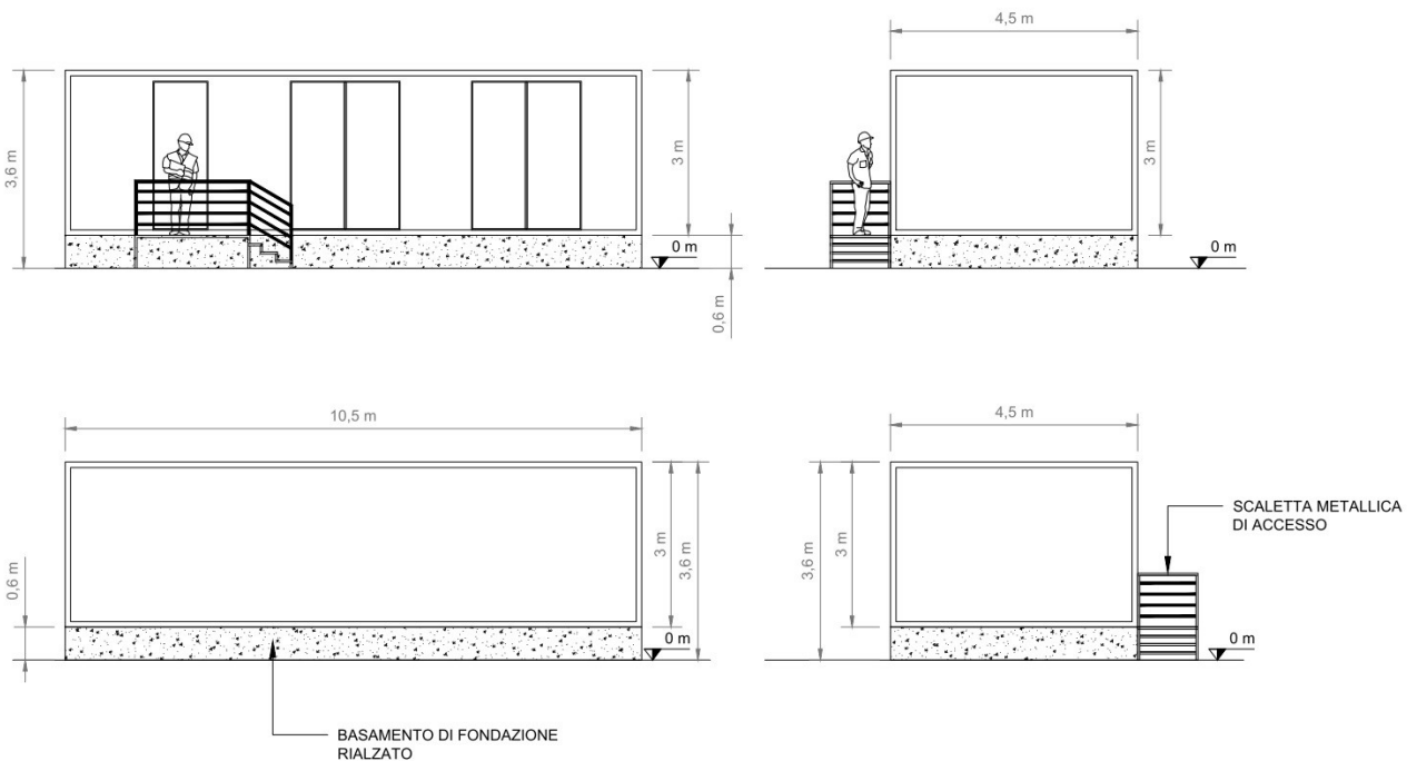
Illustrazione 3: Shelter prefabbricato metallico – prospetti e sezioni
