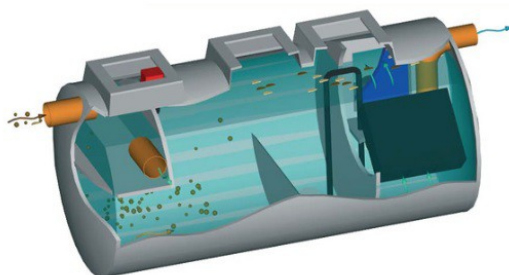
Illustrazione 4: Disoleatore
