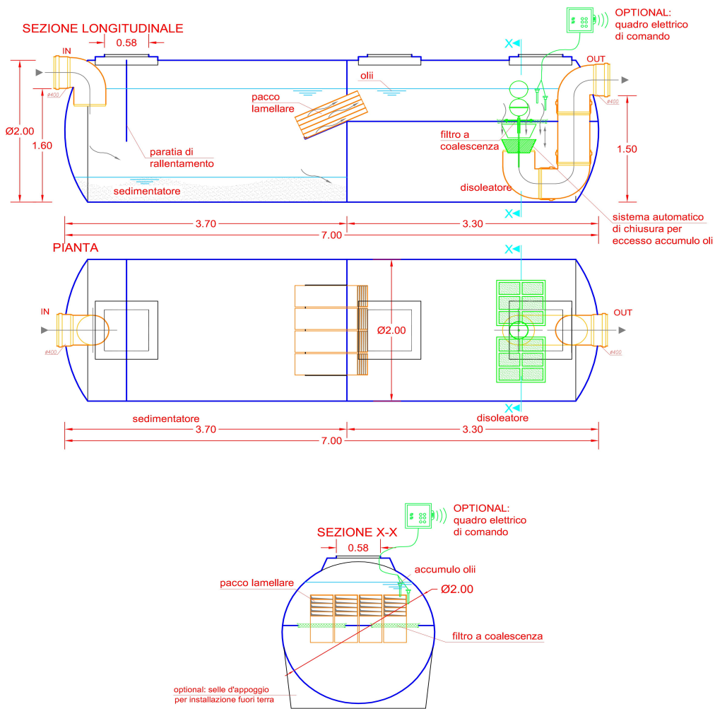
Illustrazione 5: Dimensioni disoleatore da 5 metri cubi
