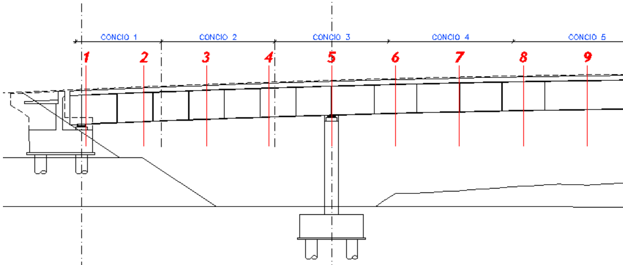
FIGURA 28 SUDDIVISIONE DELLE TRAVI IN CONCI
