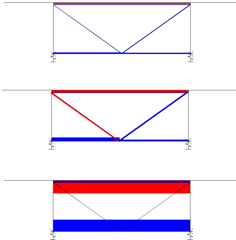
FIGURA 22 DIAGRAMMI AZIONE ASSIALE DEI DIAFRAMMI RETICOLARI
