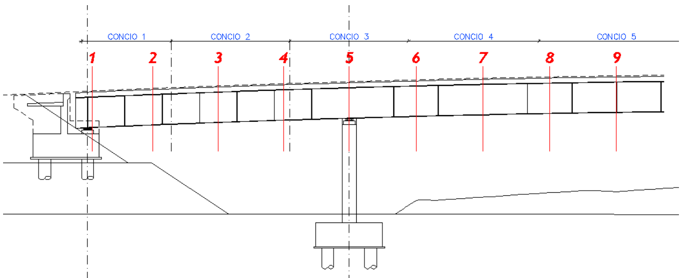
FIGURA 21 PROSPETTO DEL PONTE CON EVIDENZIATE LE SEZIONI DI ANALISI
