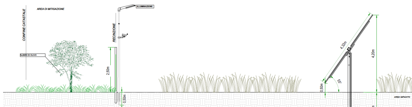
Figura-4: Sezione tipo della fascia perimetrale di mitigazione
