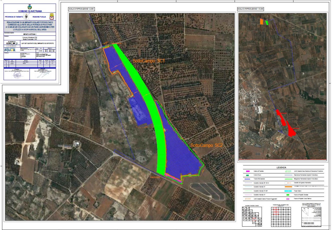
Figura 15-1: Ortofoto con vista dell'impianto fotovoltaico
