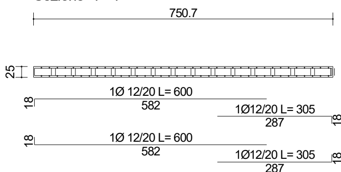
Sezione 1 - 1
