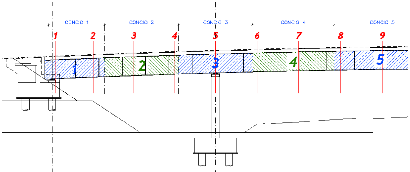
FIGURA 28 SUDDIVISIONE DELLE TRAVI IN CONCI
