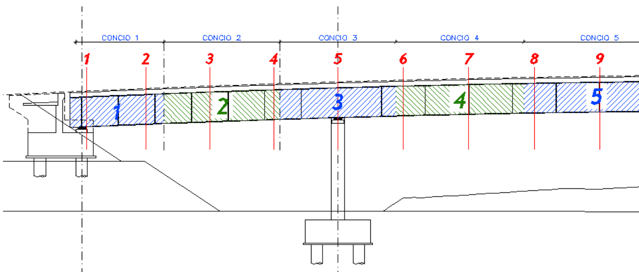
FIGURA 21 PROSPETTO DEL PONTE CON EVIDENZIATE LE SEZIONI DI ANALISI
