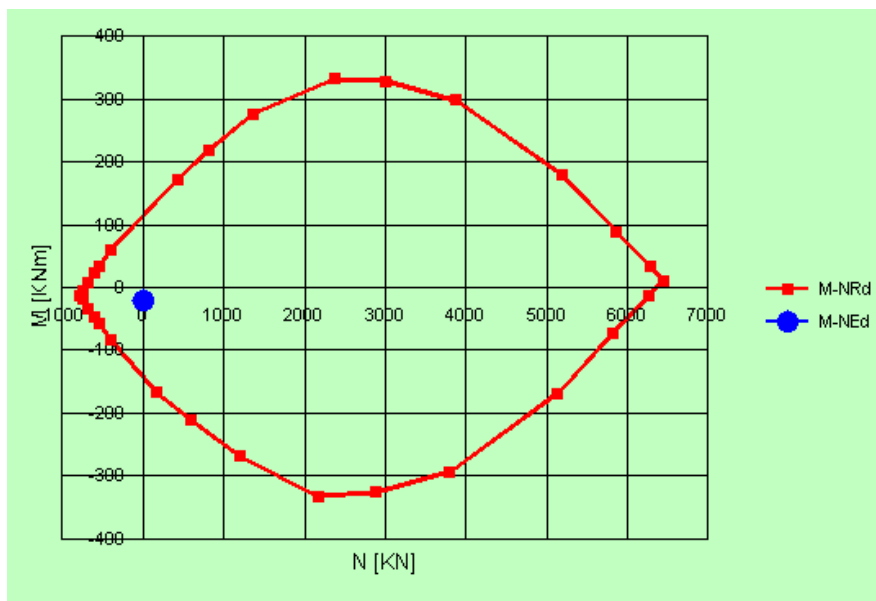
FIGURA 25 DOMINIO RESISTENTE SEZIONE LONGITUDINALE ATTACCO DELLA SBALZO
