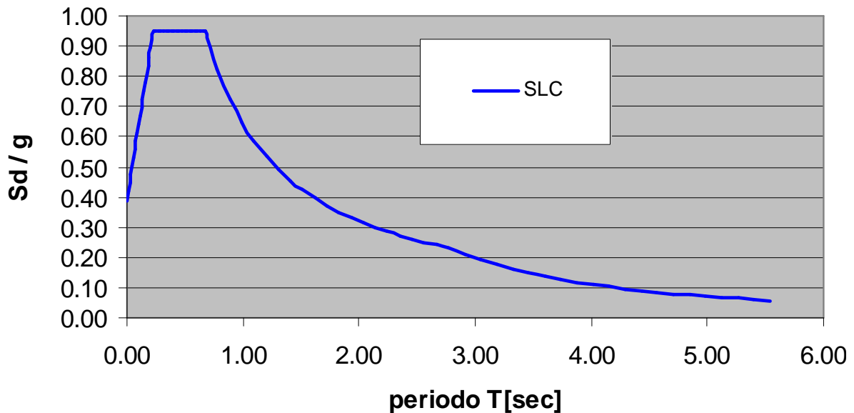
FIGURA 12 SPETTRO DI RISPOSTA ELASTICO – ACCELERAZIONE ORIZZONTALE ALLO SLC
