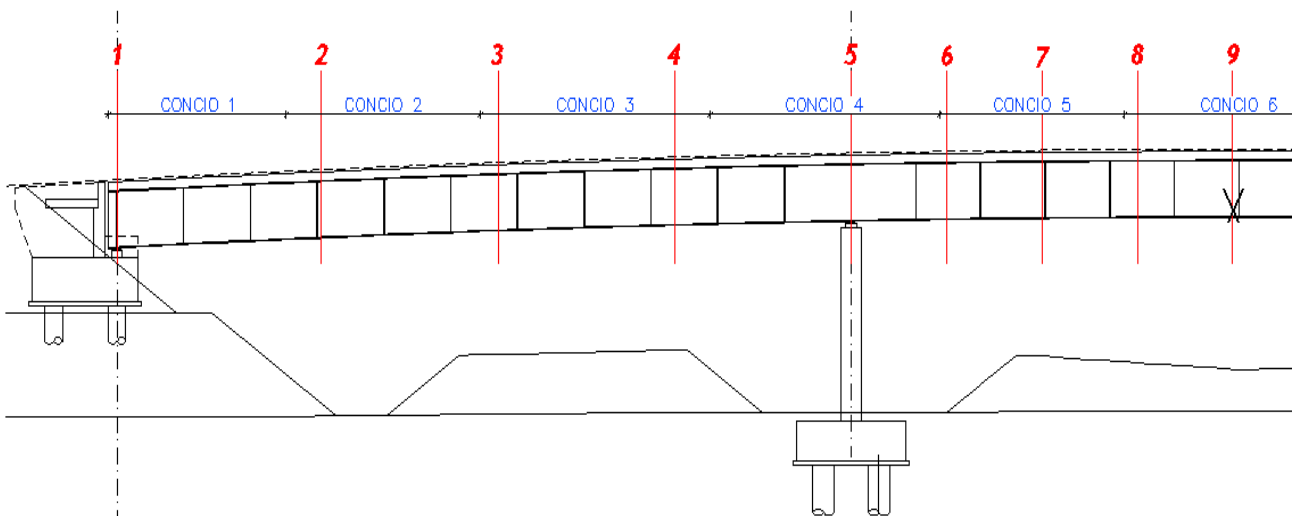
FIGURA 28 SUDDIVISIONE DELLE TRAVI IN CONCI
