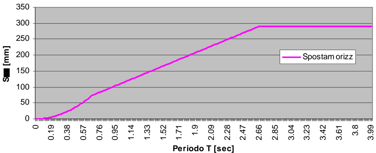
FIGURA 14 SPETTRO DI RISPOSTA IN SPOSTAMENTO ORIZZONTALE ALLO SLV
