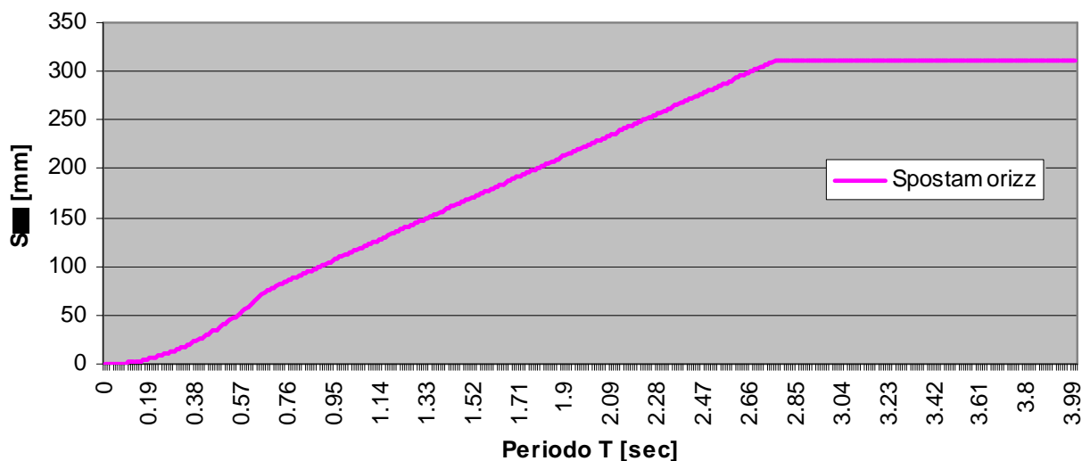
FIGURA 15 SPETTRO DI RISPOSTA IN SPOSTAMENTO ORIZZONTALE ALLO SLC
