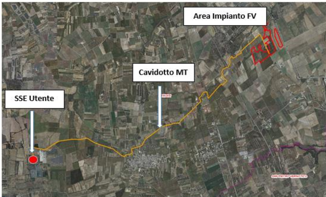
Inquadramento generale su Ortofoto – area impianto e SSE (in rosso), cavidotto MT esterno (in giallo)
