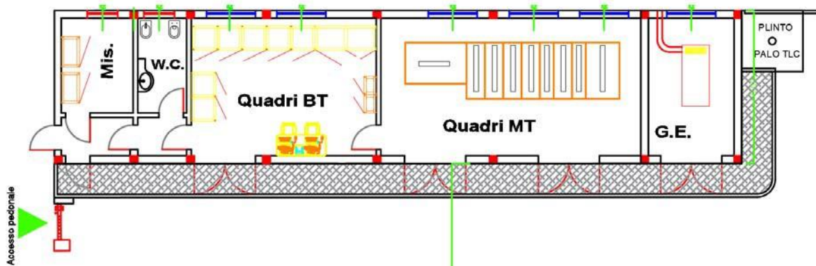
FIGURA 2: LAYOUT DELLA SSE
