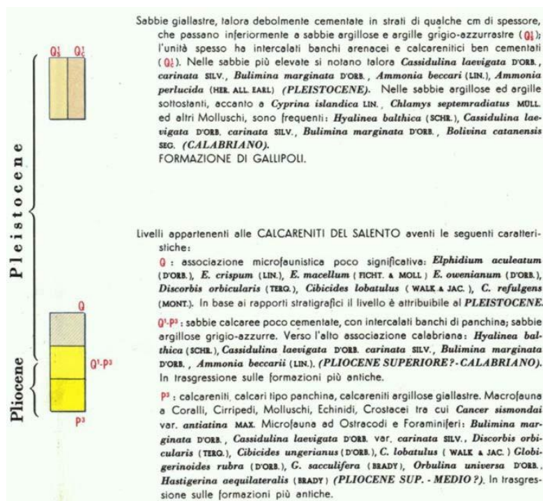
FIGURA 6: STRALCIO DELLA CARTA GEOLOGICA D'ITALIA – CERIGNOLA FOGLIO 175 – IN ROSSO L'AREA DI INTERESSE LE SABBIE SI RINVENGONO, CON PROBABILE PASSAGGIO GRADUALE, DEI DEPOSITI SABBIOSI DI NATURA CALCAREO-MICACEA. ESSE SONO AFFIORANTI ESTESAMENTE SU TUTTA L'AREA INDAGATA.
