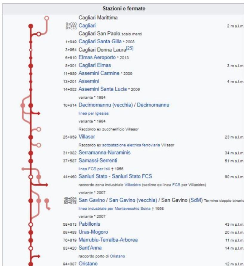
Figura 1 schematico di linea
