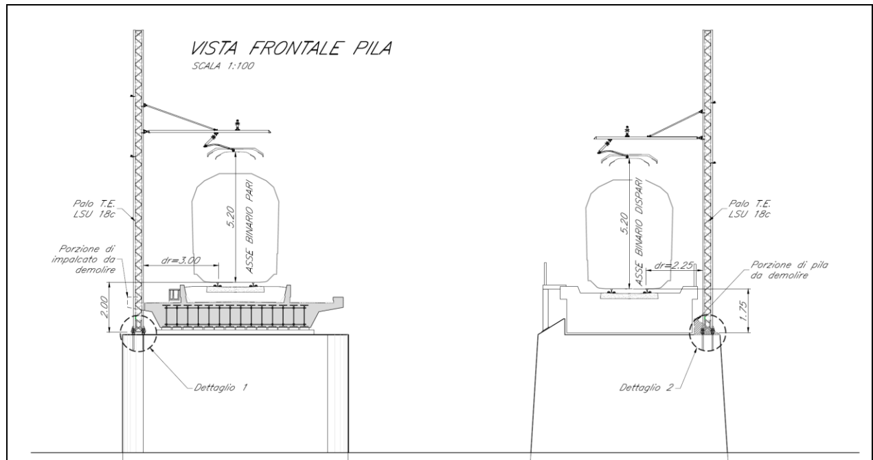
Figura 41 gli ancoraggi del Ponte km 19+340
