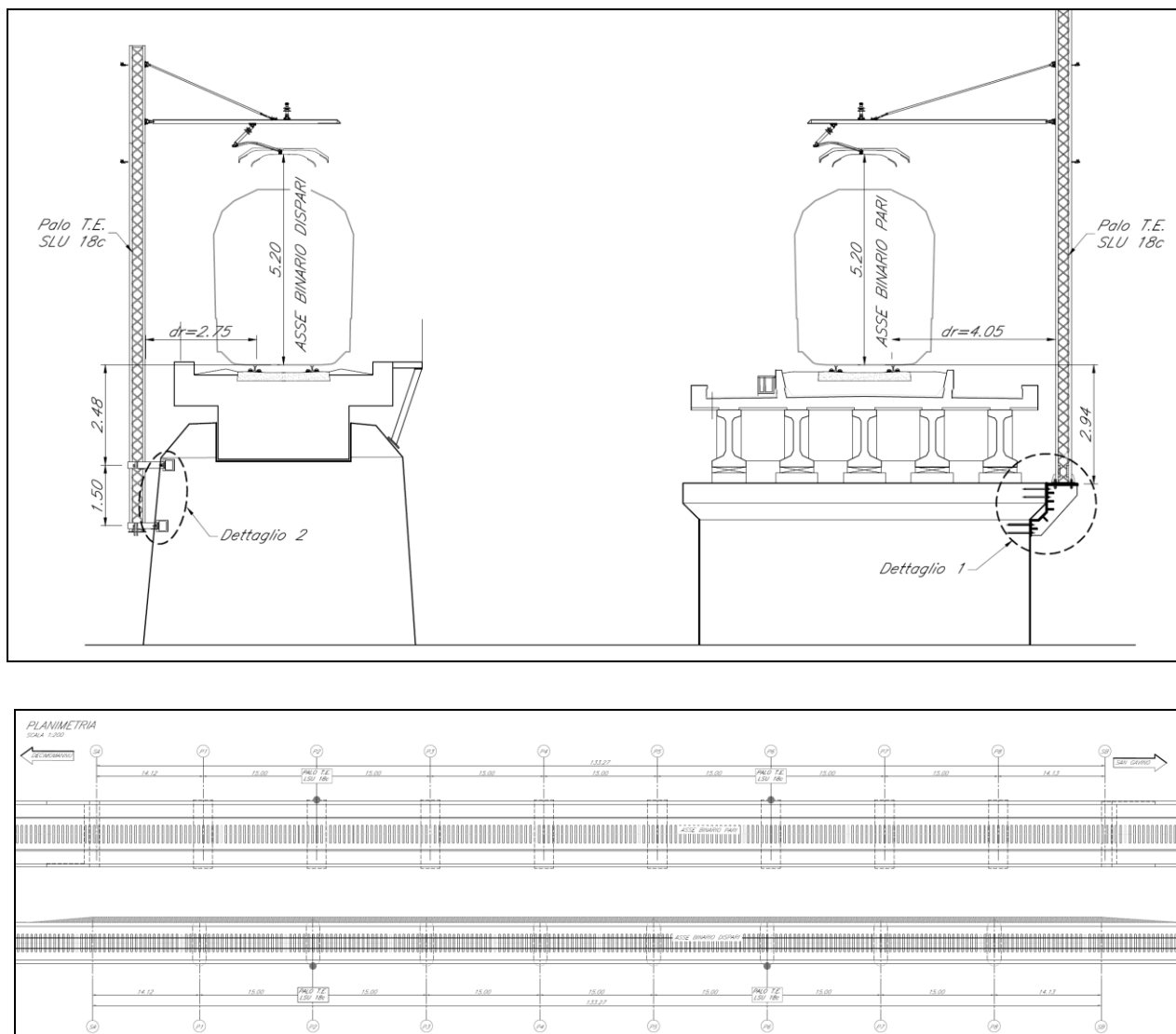
Figura 45 gli ancoraggi del Ponte km 24+933
