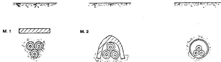
Figura 1: Modalità di posa
