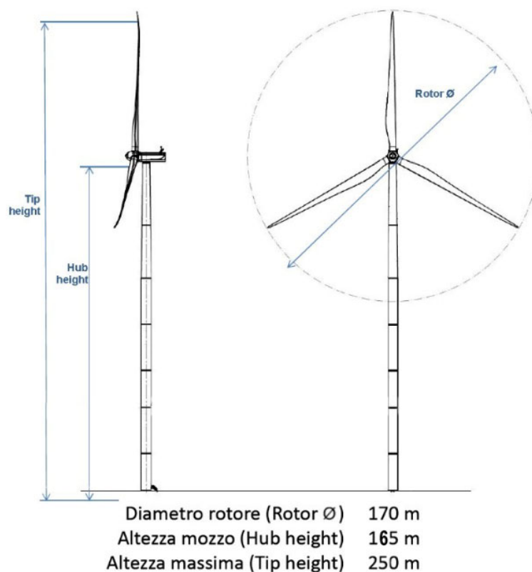
Figura 3: Vista aerogeneratore
