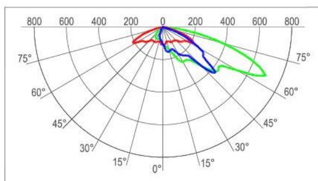
Figura 1 - curva fotometrica apparecchio utilizzato
