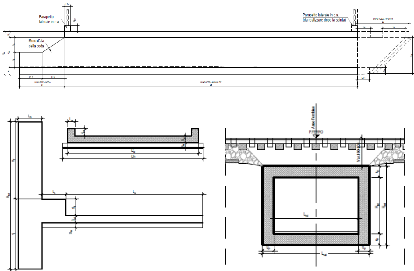
Figura 3. Geometria tipologica del monolite, della platea di varo e del muro reggispinga
