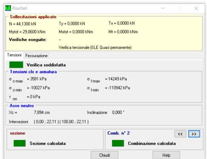
Figura 9-15 – Risultati verifica tensionale (QP).
