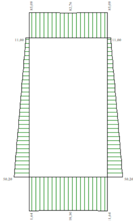
Figura 10-7 – Involuppo sforzo normale (SLU).
