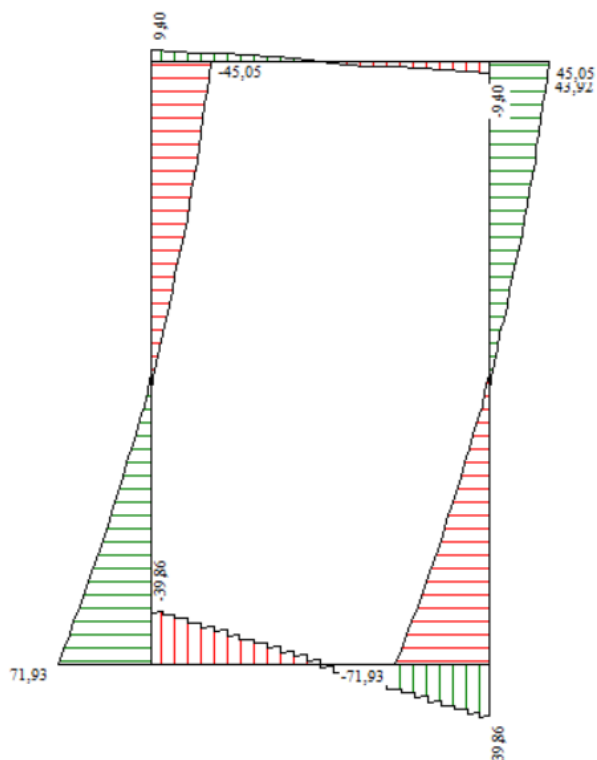
Figura 10-6 – Inviluppo taglio (SLE).
