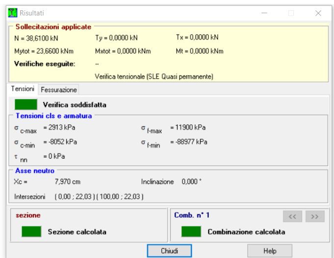
Figura 10-15 – Risultati verifica tensionale (QP).
