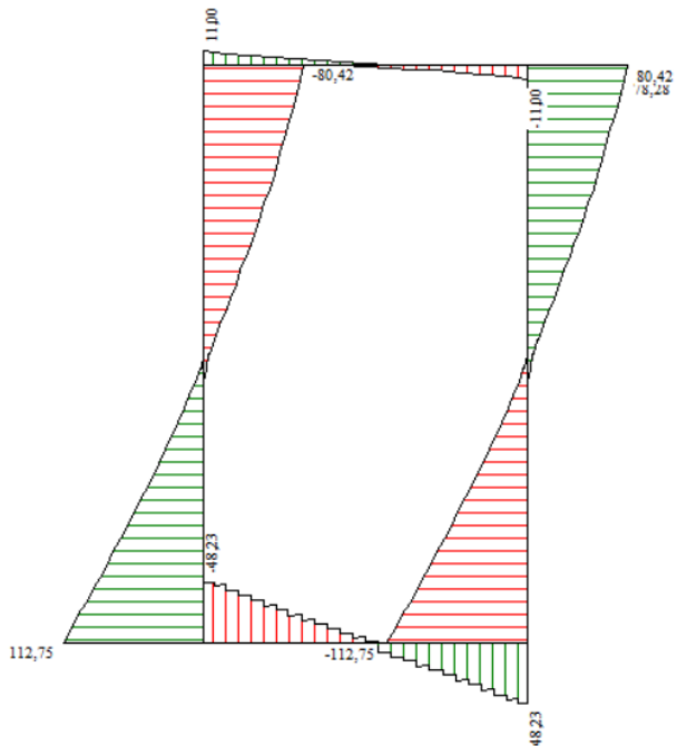
Figura 10-5 – Inviluppo taglio (SLU).
