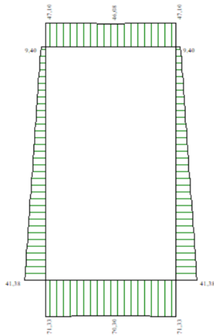
Figura 10-8 – Involuppo sforzo normale (SLE).
