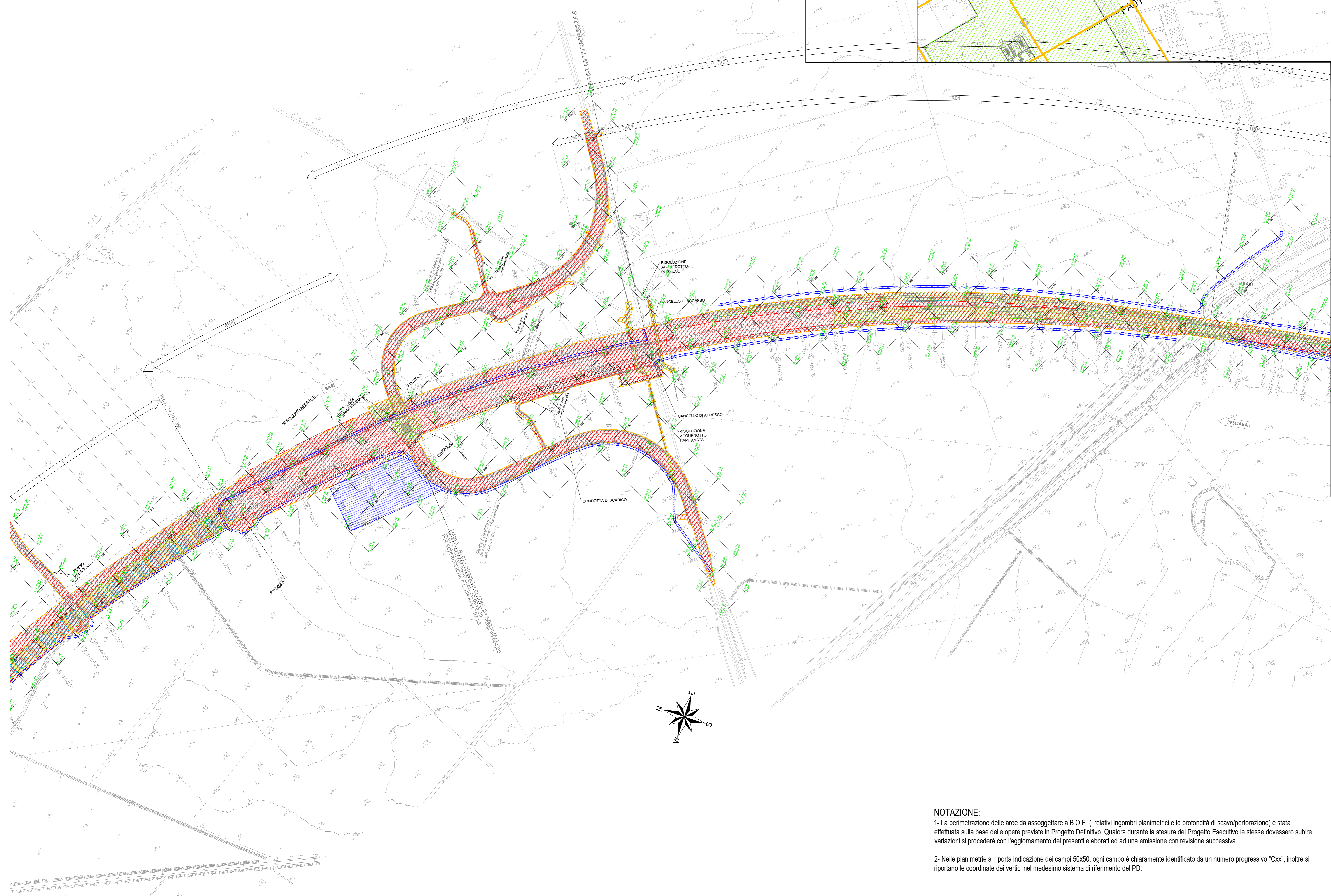
Schema bonifica da ordigni bellici profonda
