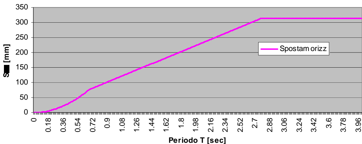
FIGURA 15 SPETTRO DI RISPOSTA IN SPOSTAMENTO ORIZZONTALE ALLO SLC
