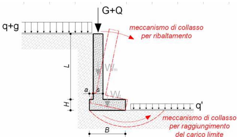
FIGURA 23 SCHEMA DELLE AZIONI
