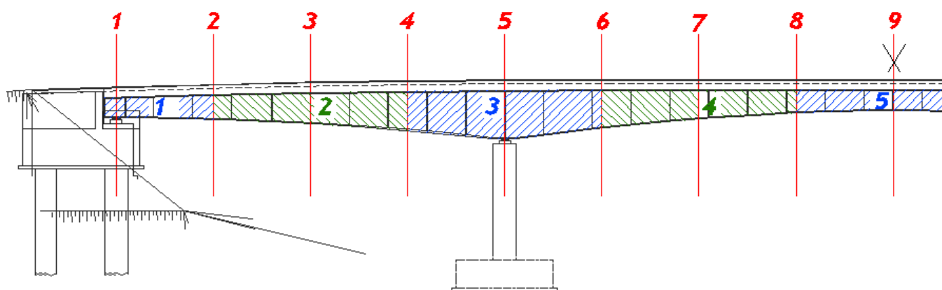
FIGURA 28 SUDDIVISIONE DELLE TRAVI IN CONCI
