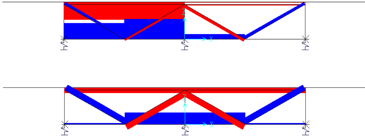
FIGURA 22 DIAGRAMMI AZIONE ASSIALE DEI DIAFRAMMI RETICOLARI
