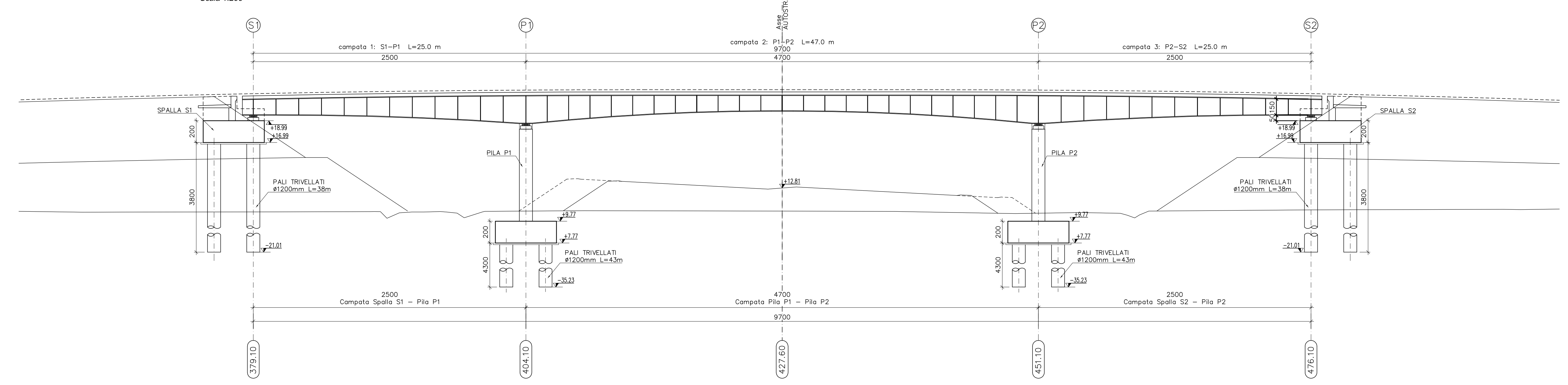
SOTTOSTRUTTURE E FONDAZIONI - SEZIONE LONGITUDINALE Scala 1:200
