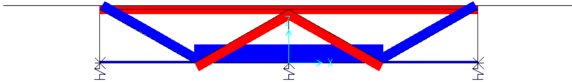
FIGURA 22 DIAGRAMMI AZIONE ASSIALE DEI DIAFRAMMI RETICOLARI
