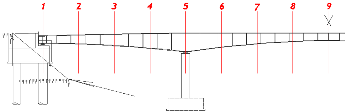
FIGURA 21 PROSPETTO DEL PONTE CON EVIDENZIATE LE SEZIONI DI ANALISI
