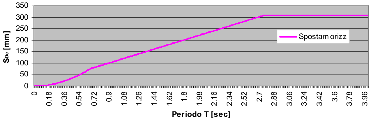
FIGURA 15 SPETTRO DI RISPOSTA IN SPOSTAMENTO ORIZZONTALE ALLO SLC
