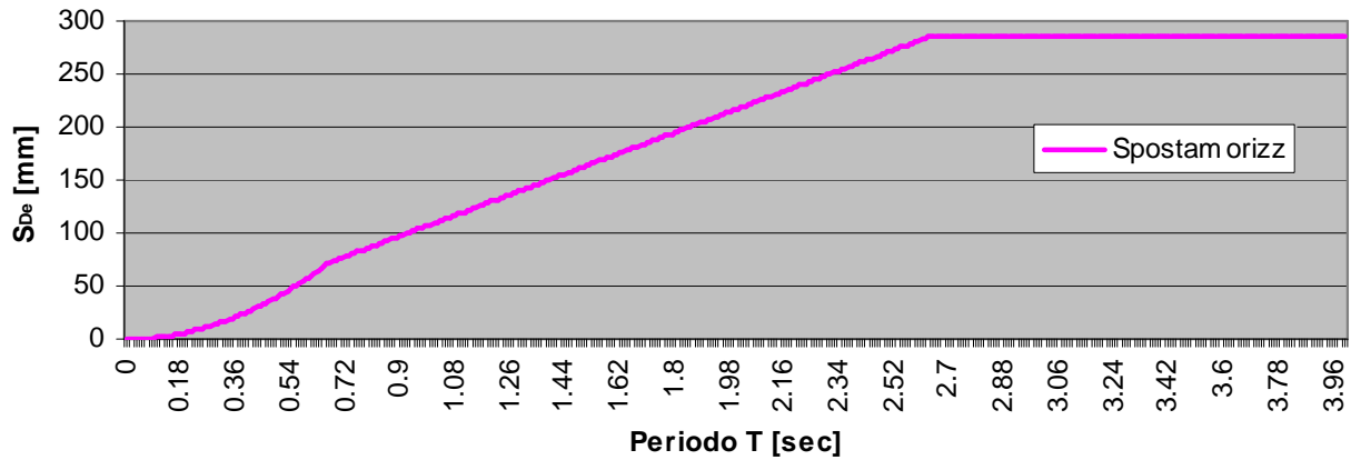
FIGURA 14 SPETTRO DI RISPOSTA IN SPOSTAMENTO ORIZZONTALE ALLO SLV
