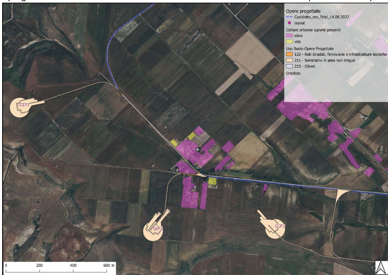
Figura 25 – Particolare della classificazione di suo del suolo, come da CTR, per gli aerogeneratori 1, 2 e 3.
