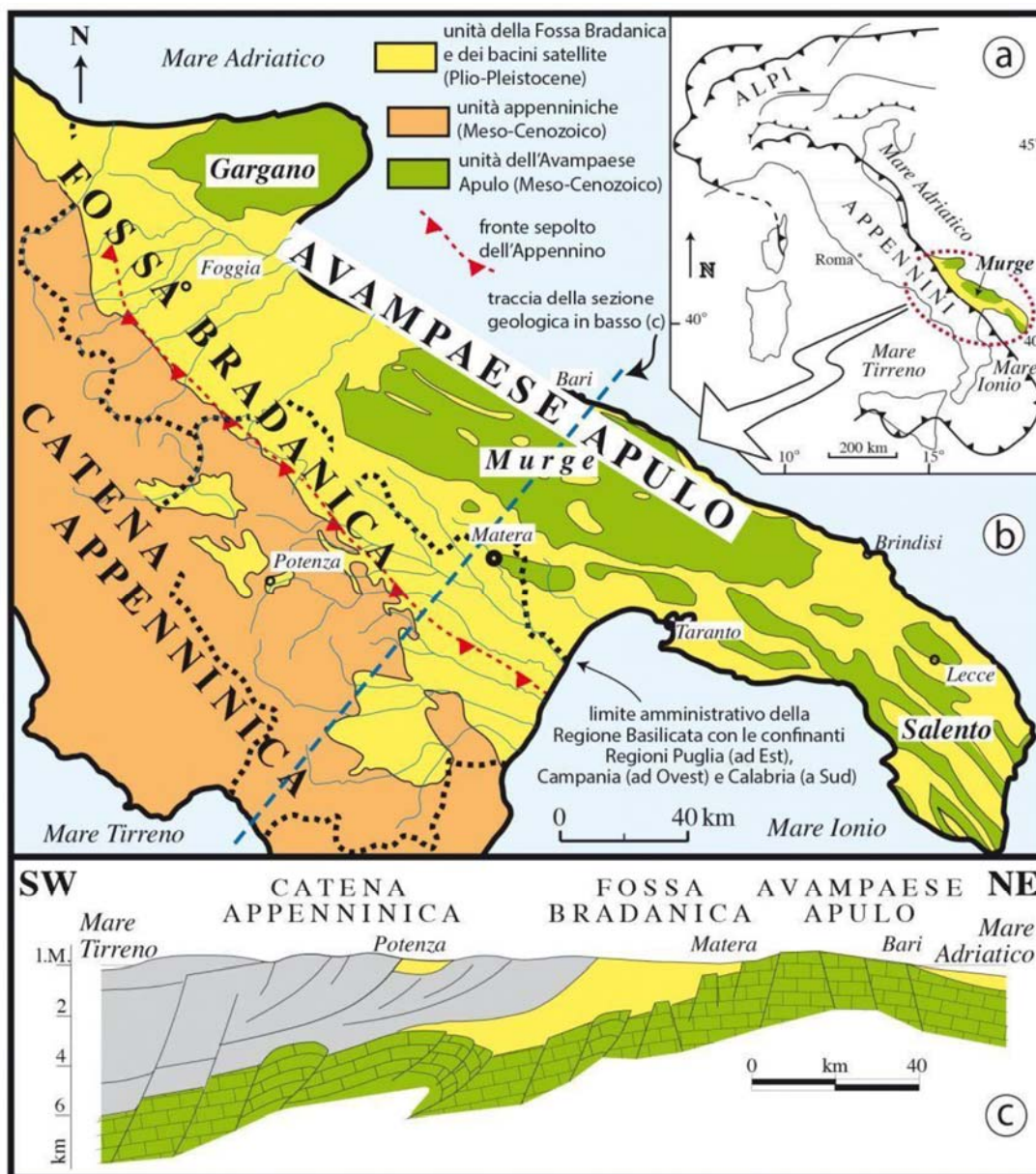
Figura 9 Carta geologica schematica della Puglia e delle aree limitrofe
