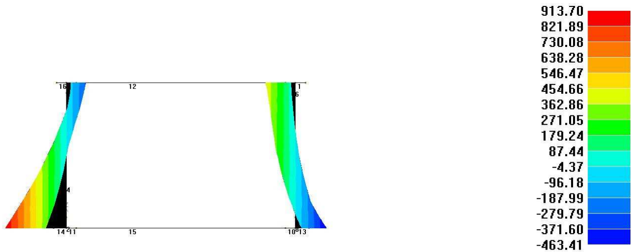
PROGETTO Inviluppo sollecitazioni Taglio 2 [kN]
