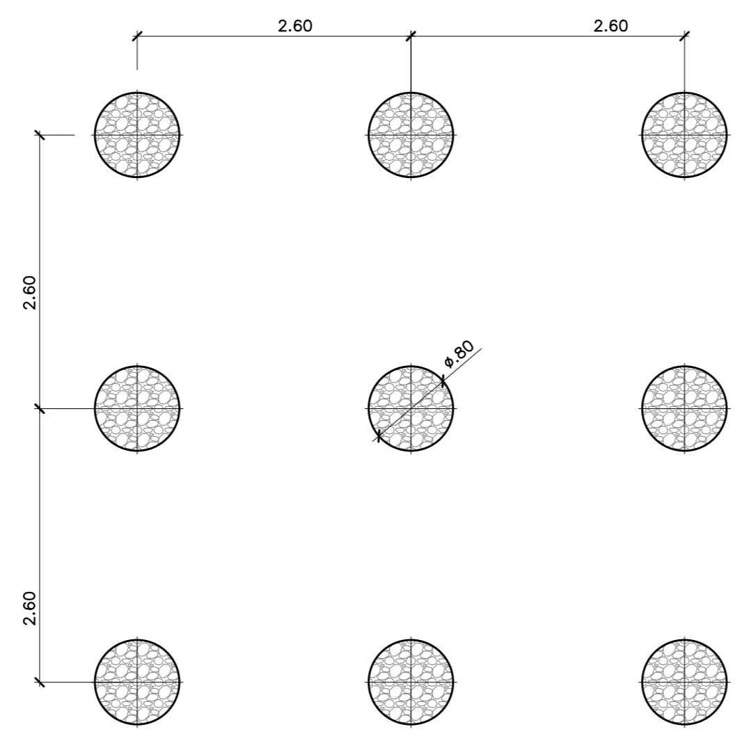
SCHEMA DI PIANTA DEL CONSOLIDAMENTO INCLUSIONI RIGIDE SCALA 1:50
