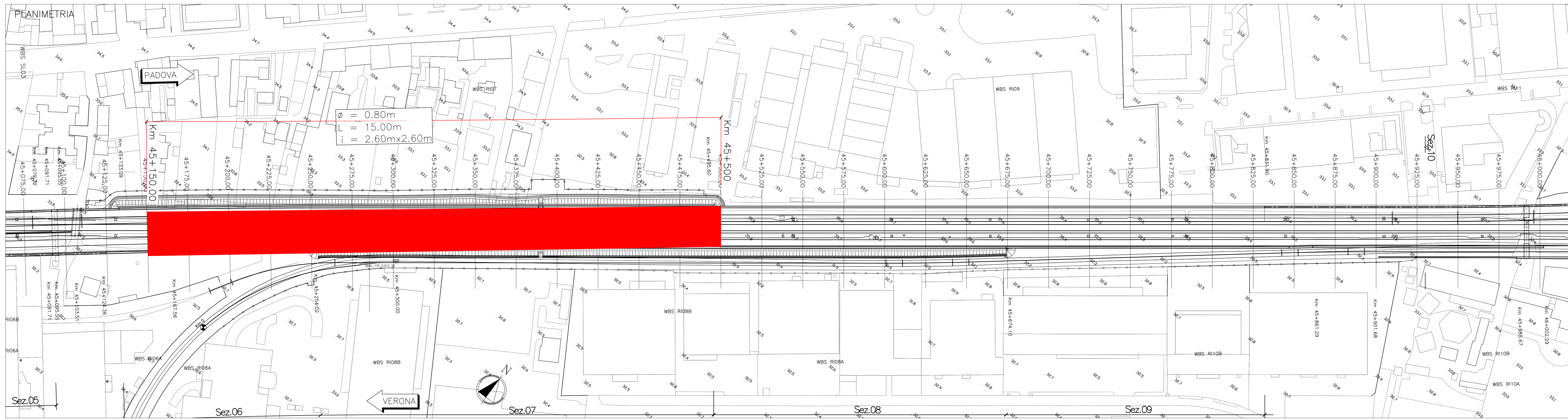
SCHEMA DI PIANTA DEL CONSOLIDAMENTO INCLUSIONI RIGIDE SCALA 1:50
