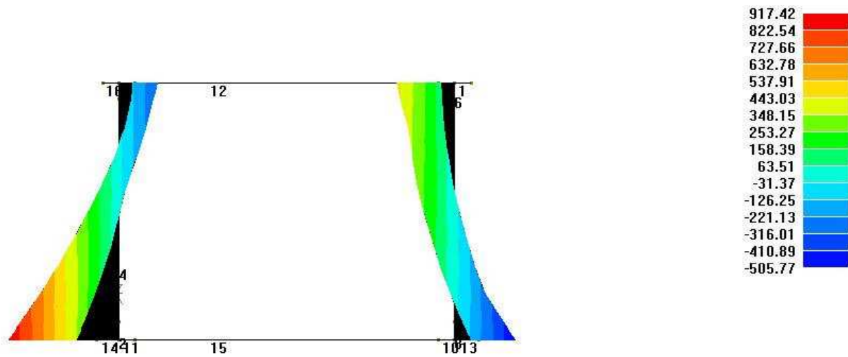
PROGETTO Inviluppo sollecitazioni Taglio 2 [kN]
