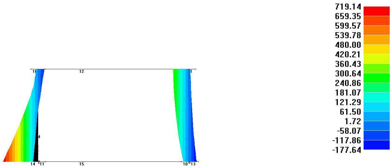
PROGETTO Involuppo sollecitazioni Taglio 2 [kN]
