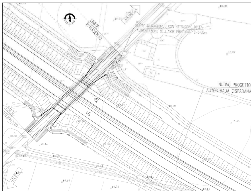
FIGURA 1.1 – SCHEMA PLANIMETRICO
