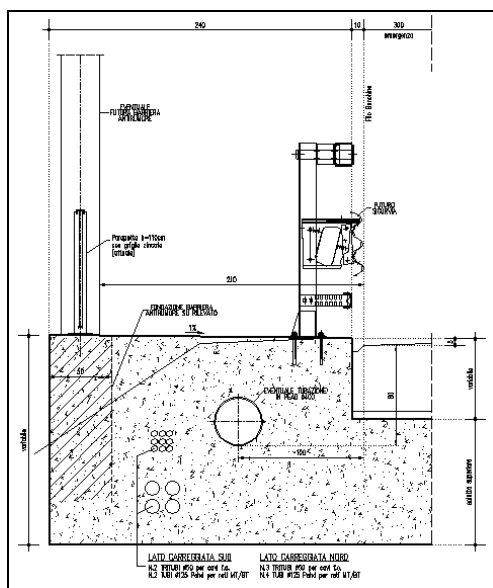
FIGURA 3.1.2 – PARTICOLARE CORDOLO AUTOSTRADALE SUL SOTTOVIA
