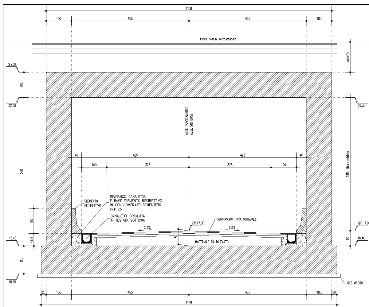
FIGURA 3.1.1 – SEZIONE TRASVERSALE DEL SOTTOVIA
