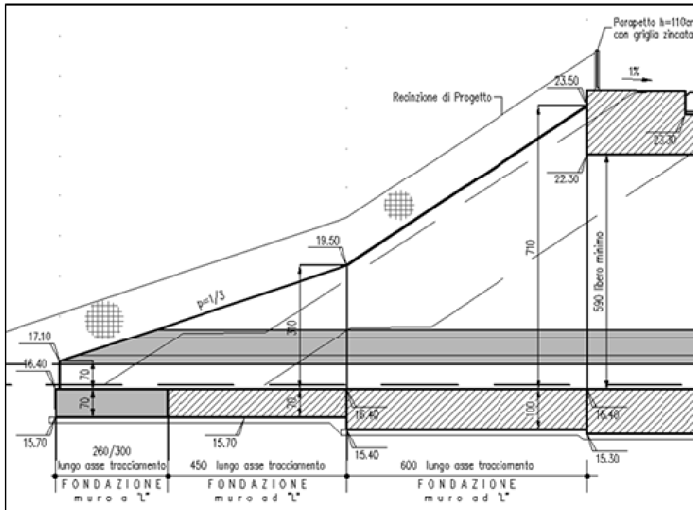
FIGURA 3.2.1 – PARTICOLARE IMBOCCO SOTTOVIA
