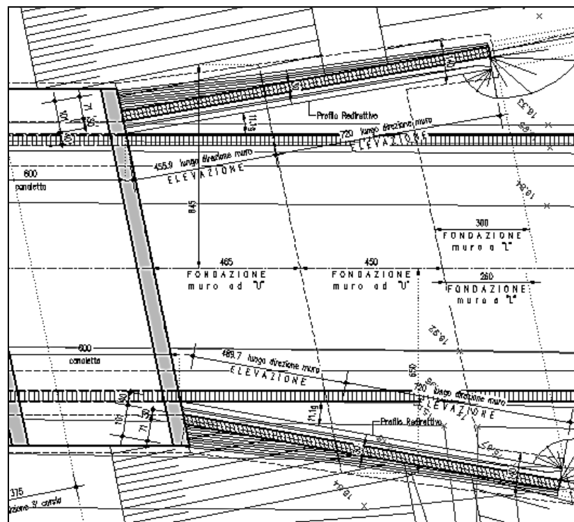
FIGURA 3.2.2 – PARTICOLARE ALLARGAMENTO PLANIMETRICO DELLE ELEVAZIONI NORD
