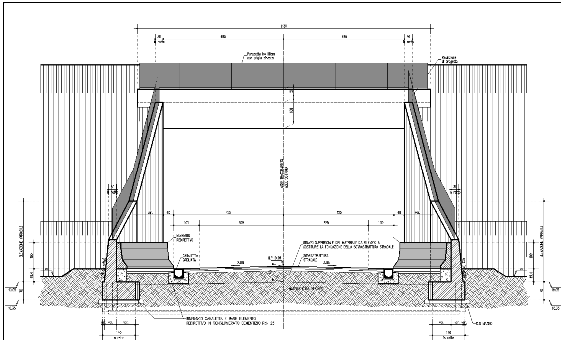
FIGURA 3.2.3 – SEZIONE TRASVERSALE SUI MURI DI IMBOCCO AD “L”
