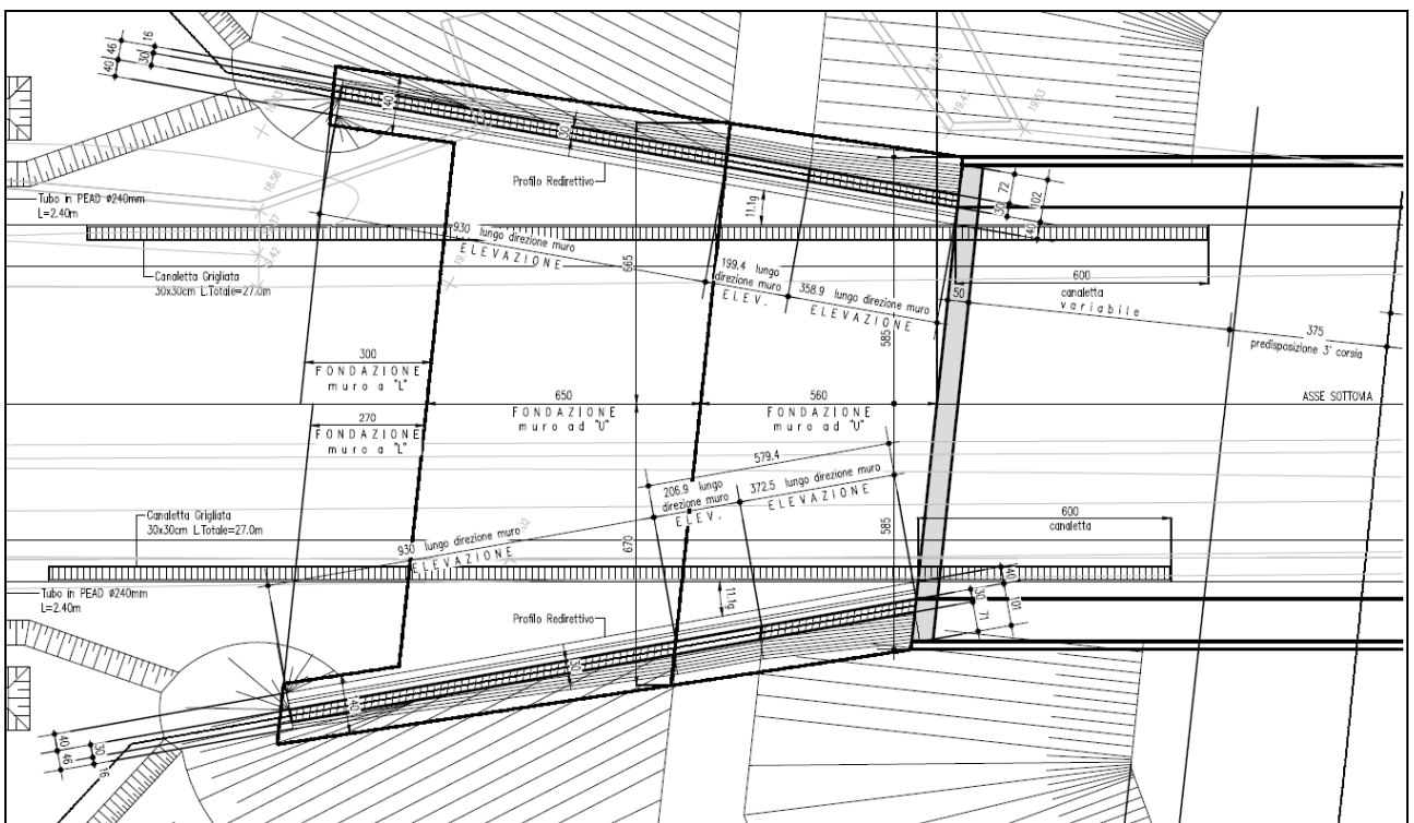
FIGURA 3.2.2 – PARTICOLARE ALLARGAMENTO PLANIMETRICO DELLE ELEVAZIONI
