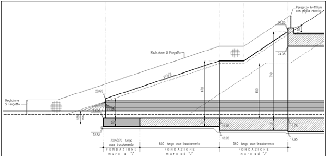
FIGURA 3.2.1 – PARTICOLARE IMBOCCO SOTTOVIA
