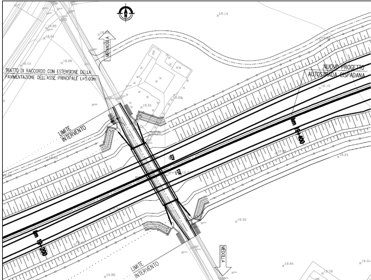
FIGURA 1.1 – SCHEMA PLANIMETRICO
