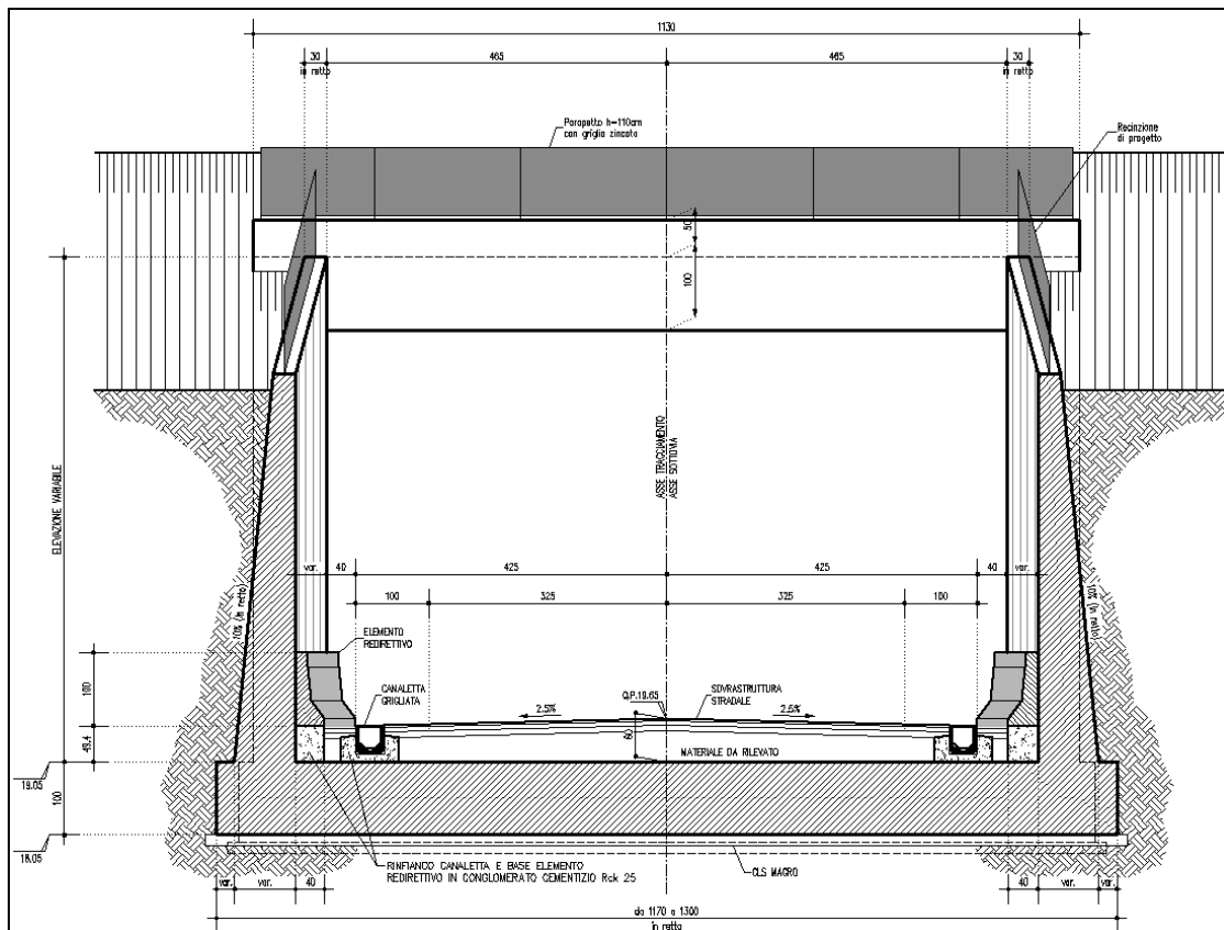
FIGURA 3.2.4 – SEZIONE TRASVERSALE SUL MURO DI IMBOCCO AD “U”
