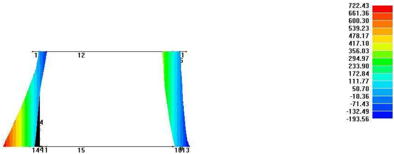
PROGETTO Involuppo sollecitazioni Taglio 2 [kN]
