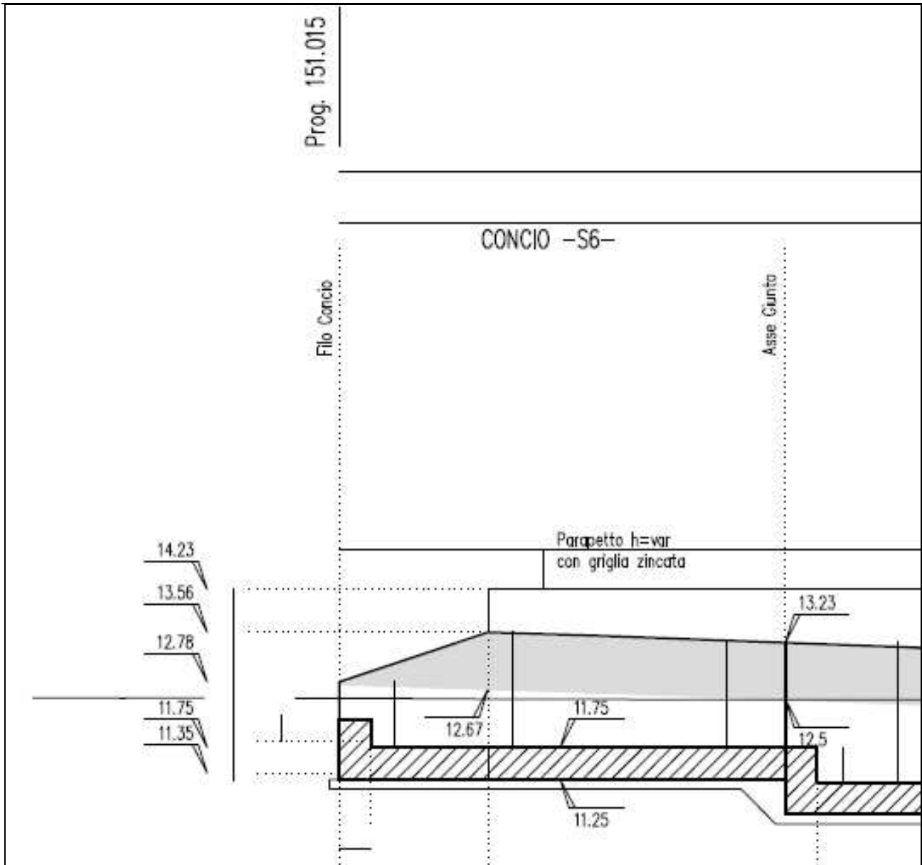
FIGURA 3.2.1 – PARTICOLARE CONCIO DI ESTREMITÀ'
