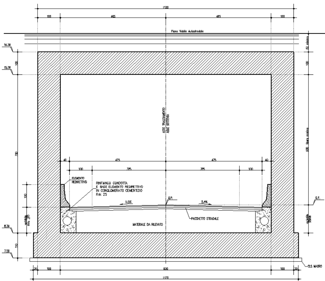
FIGURA 3.1.1 – SEZIONE TRASVERSALE DEL SOTTOVIA
