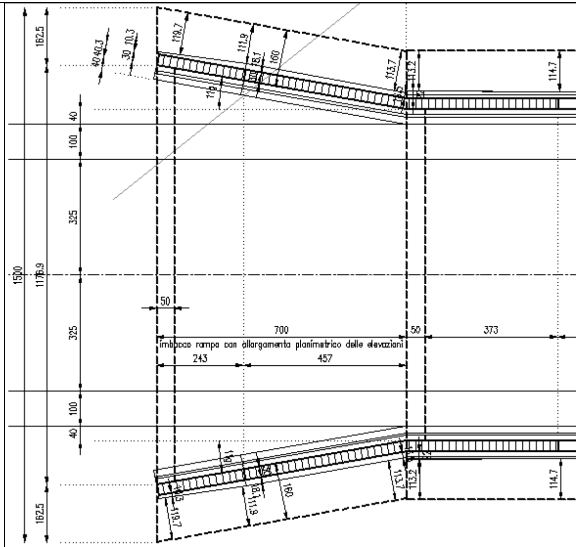
FIGURA 3.2.2 – PLANIMETRIA MURI AD U IN INGRESSO DEL SOTTOVIA S.V. GNOLA
