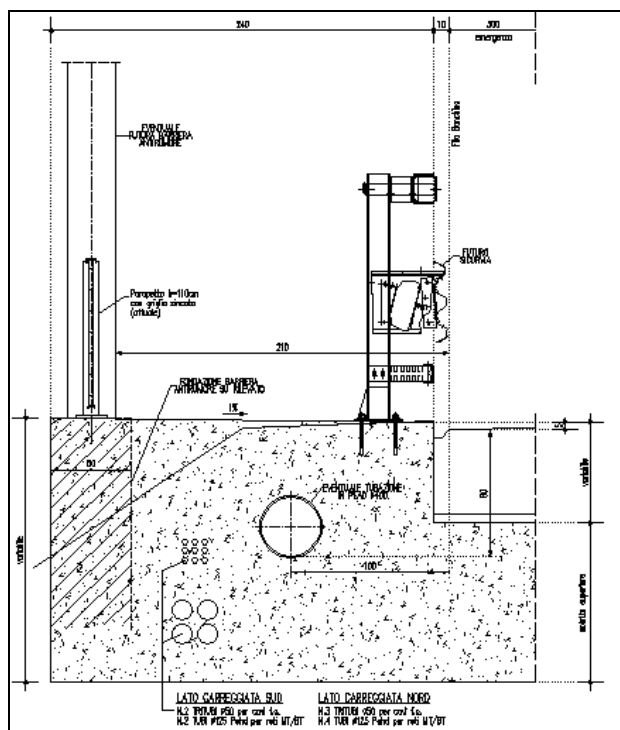
FIGURA 3.1.2 – PARTICOLARE CORDOLI AUTOSTRADALI IN PROSSIMITA' DEL SOTTOVIA
