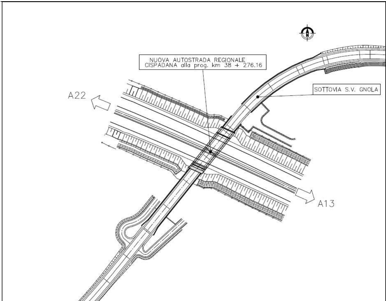
FIGURA 1-1 – SCHEMA PLANIMETRICO
