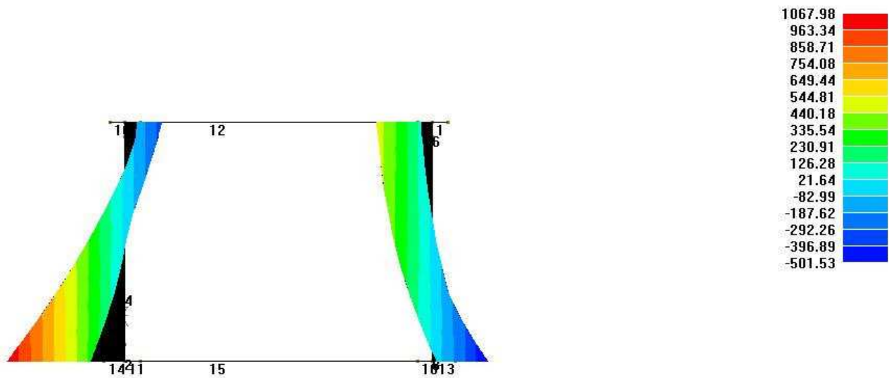
PROGETTO Inviluppo sollecitazioni Taglio 2 [kN]
