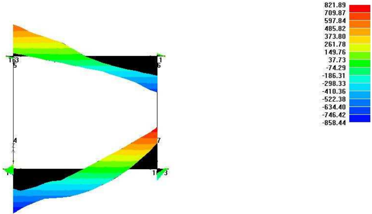
PROGETTO Inviluppo sollecitazioni Taglio 2 [kN]
