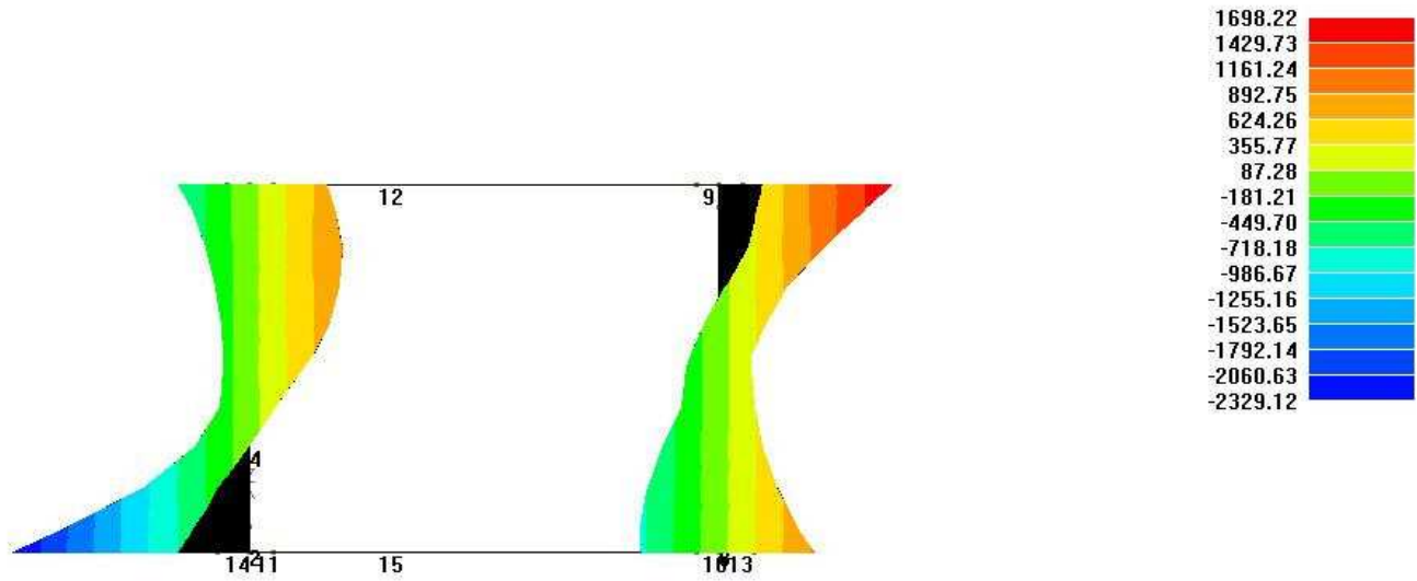
PROGETTO Inviluppo sollecitazioni Momento 3-3 [kN m]
