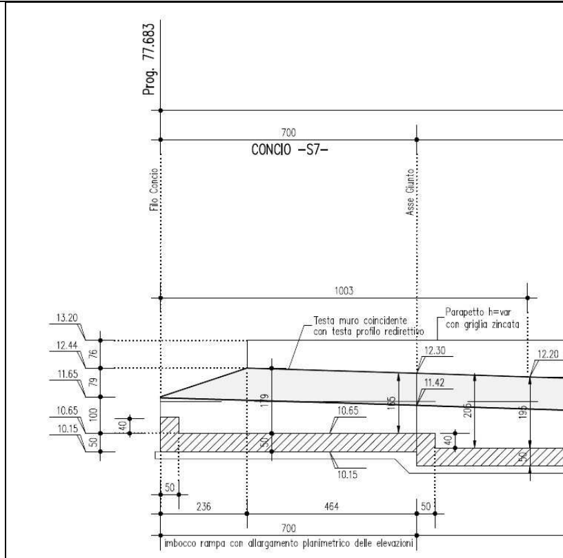
FIGURA 3.2-1 – PARTICOLARE CONCIO DI ESTREMITÀ
