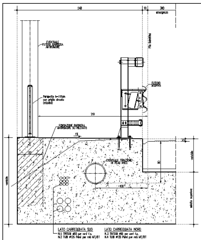
FIGURA 3.1.2 – PARTICOLARE CORDOLI AUTOSTRADALI SUL SOTTOVIA
