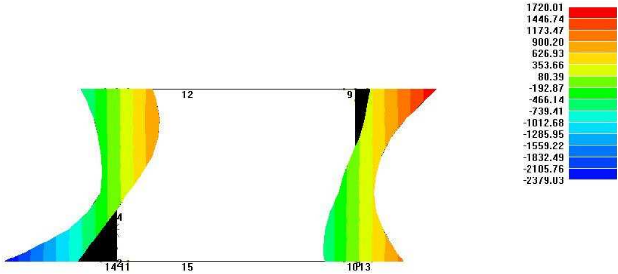
PROGETTO Inviluppo sollecitazioni Momento 3-3 [kN m]
