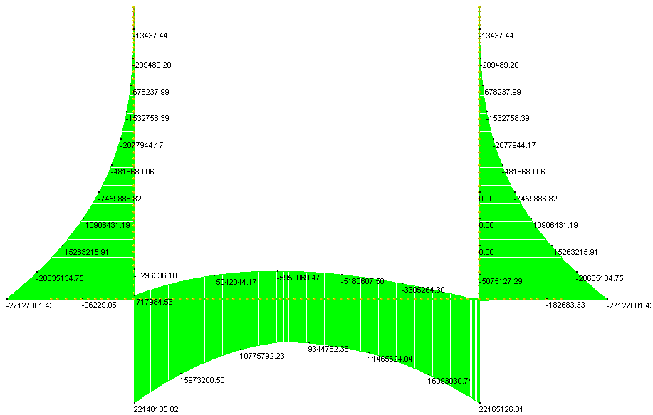
Inviluppo SLU
