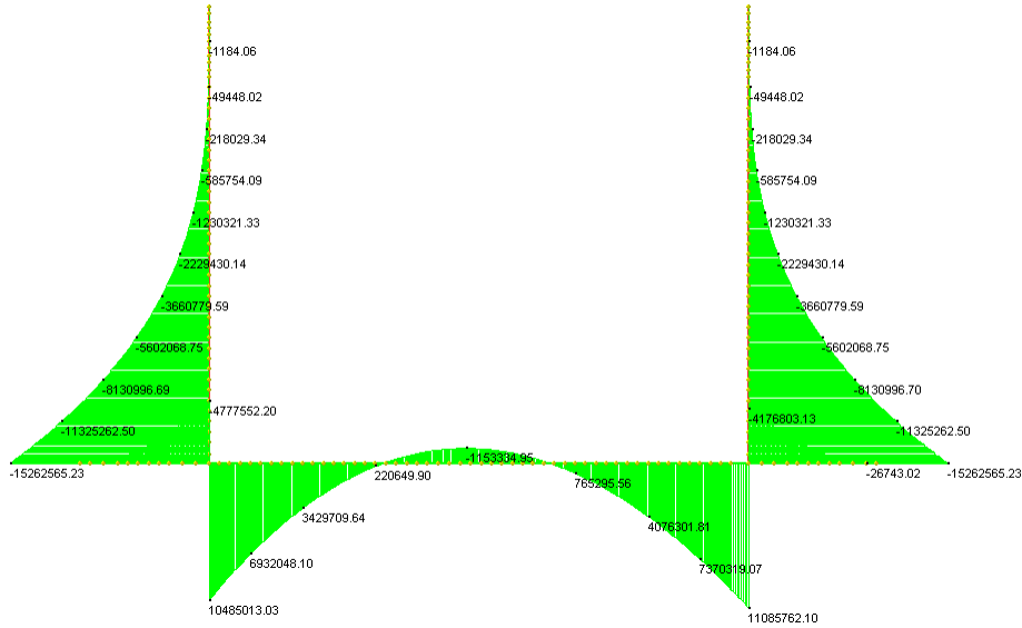
Inviluppo QUASI PERMANENTE
