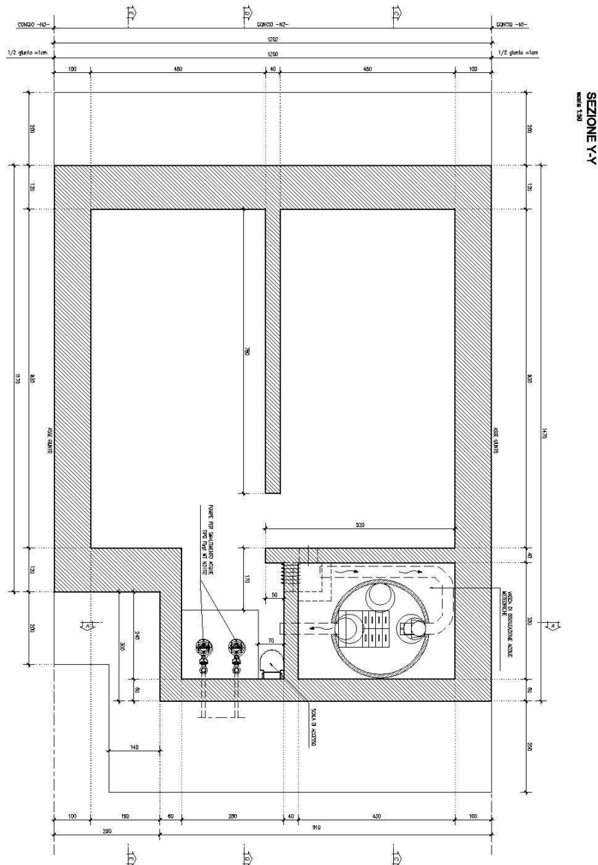
Fig. 1- Pianta vasca
