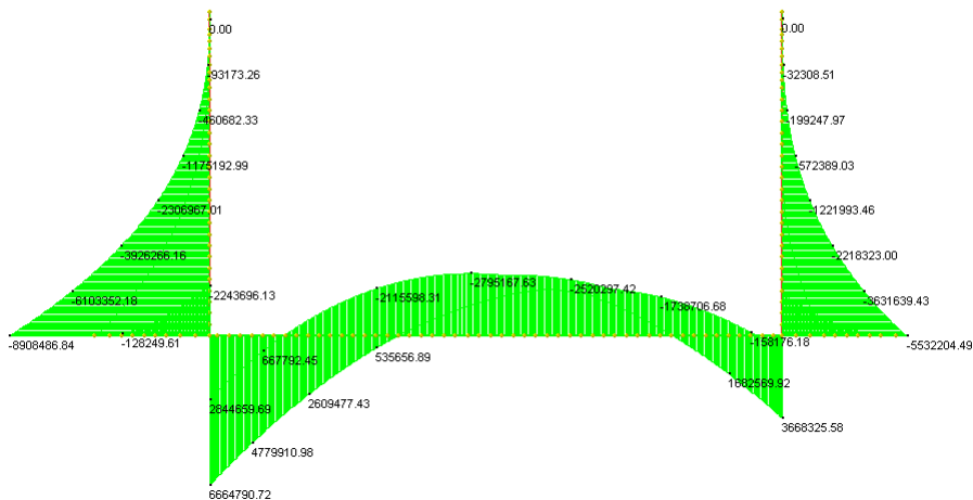
Inviluppo SLV
