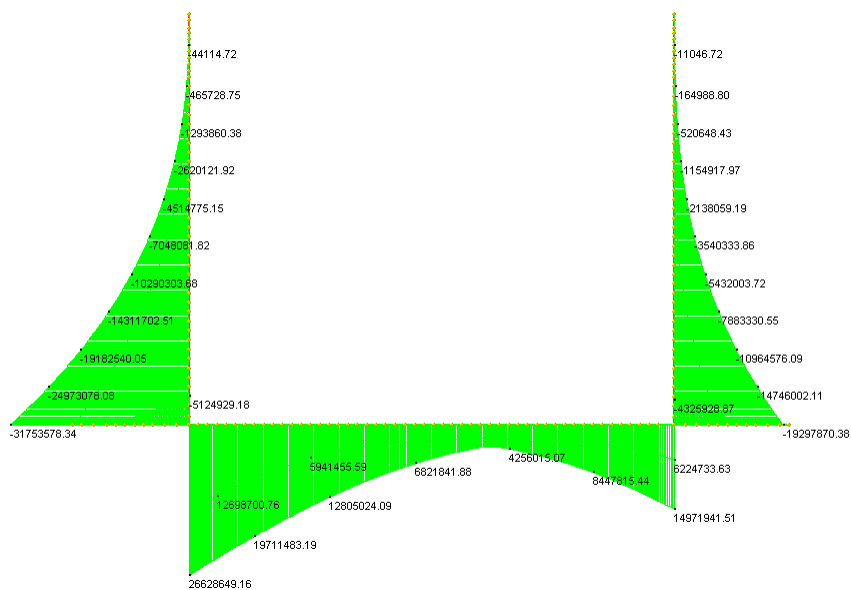
Inviluppo SLV
