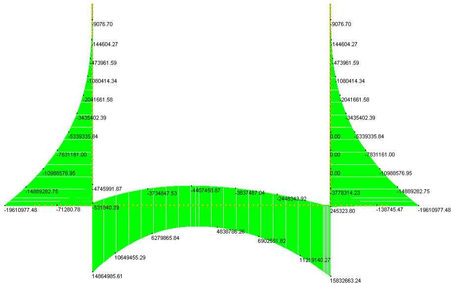
Inviluppo RARA
