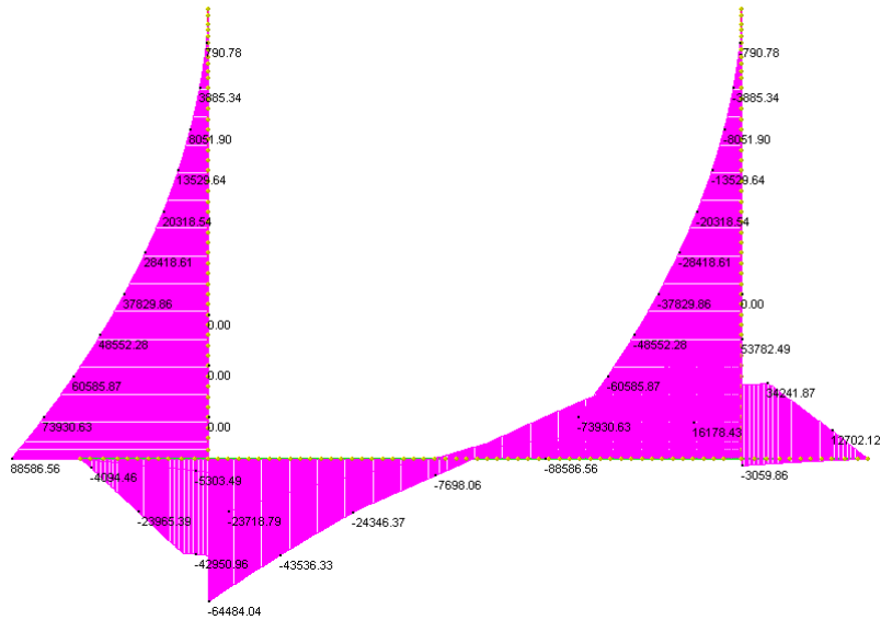
Inviluppo SLU
