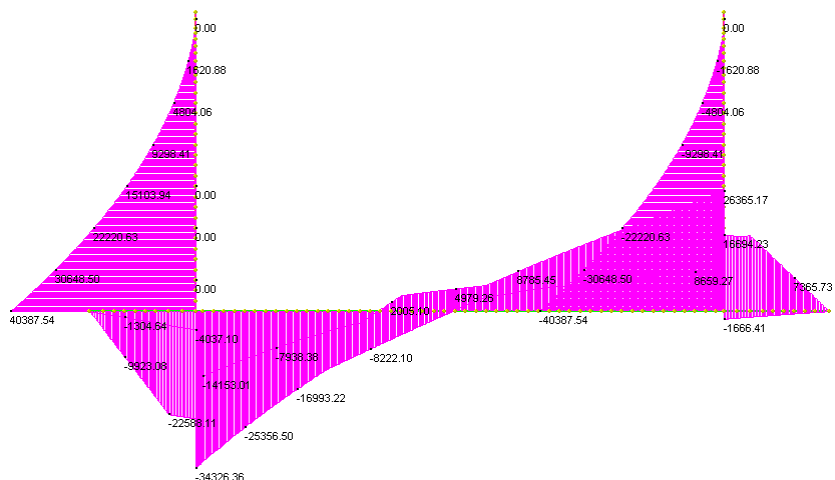
Inviluppo SLU
