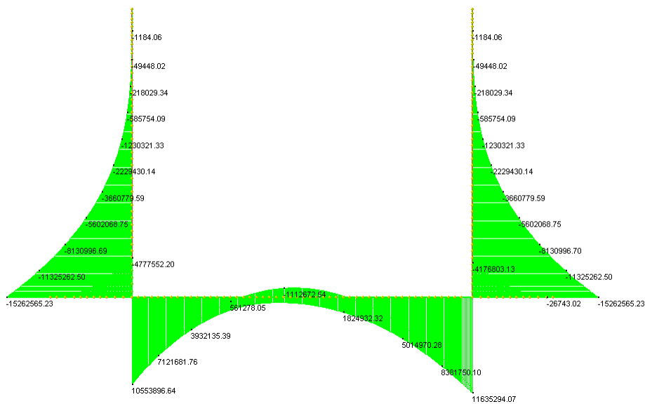
Inviluppo FREQUENTE
