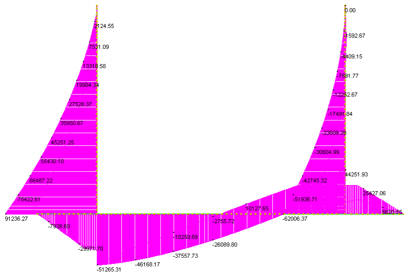
Inviluppo SLV
