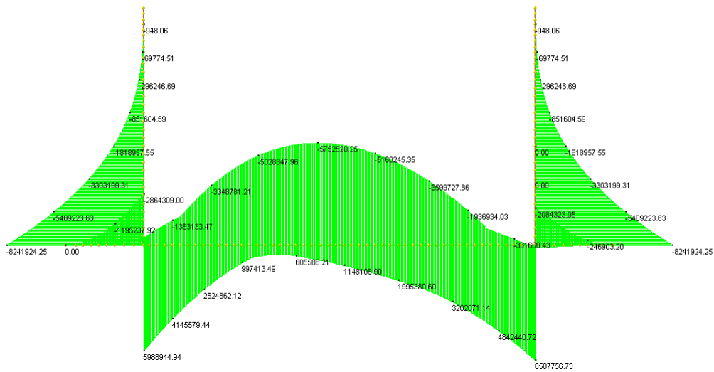
Inviluppo SLU
