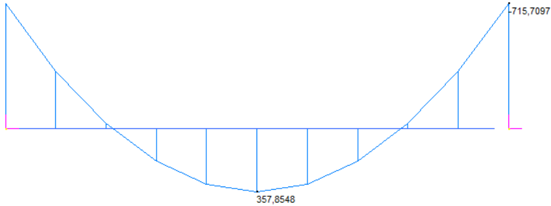
Momento SLV (fascia alta)
