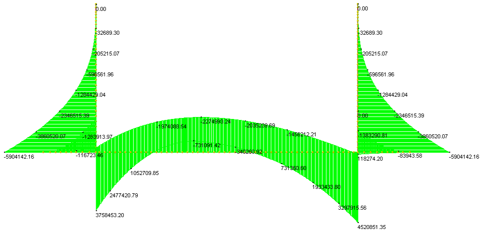
Inviluppo RARA
