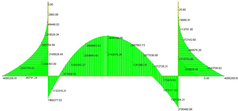
Inviluppo FREQUENTE
