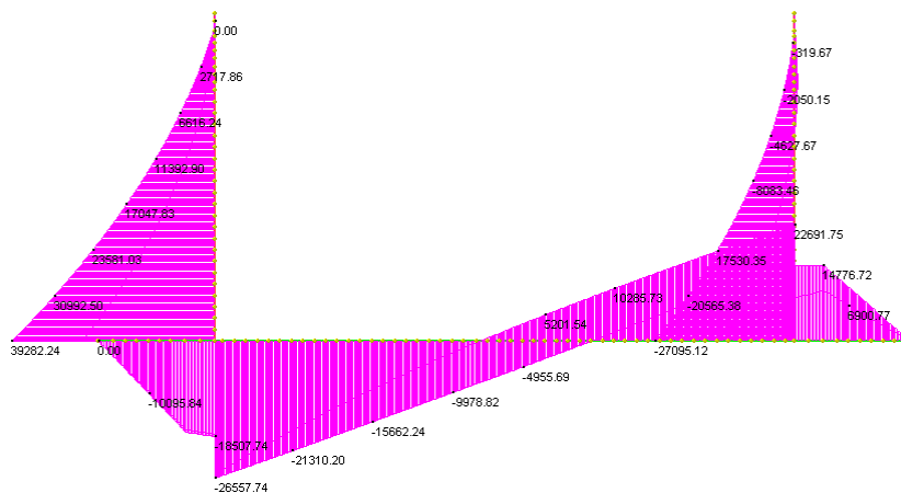
Inviluppo SLV
