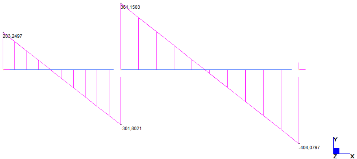
Taglio SLU (fascia bassa)
