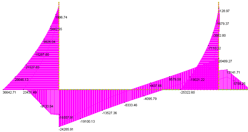
Inviluppo SLV
