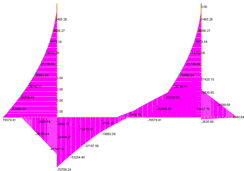
Inviluppo SLU
