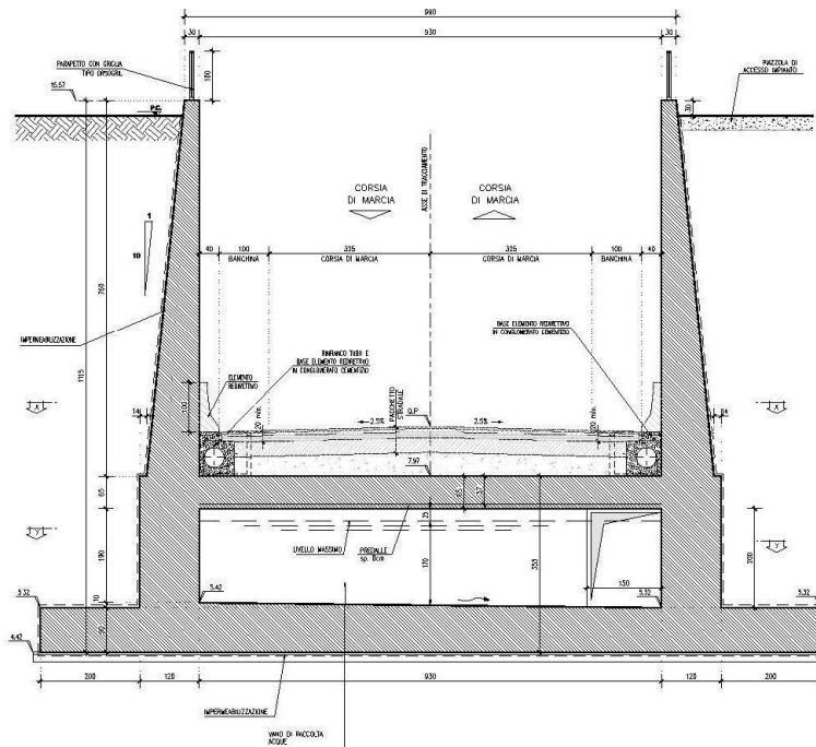
Fig. 2- Sezione verticale
