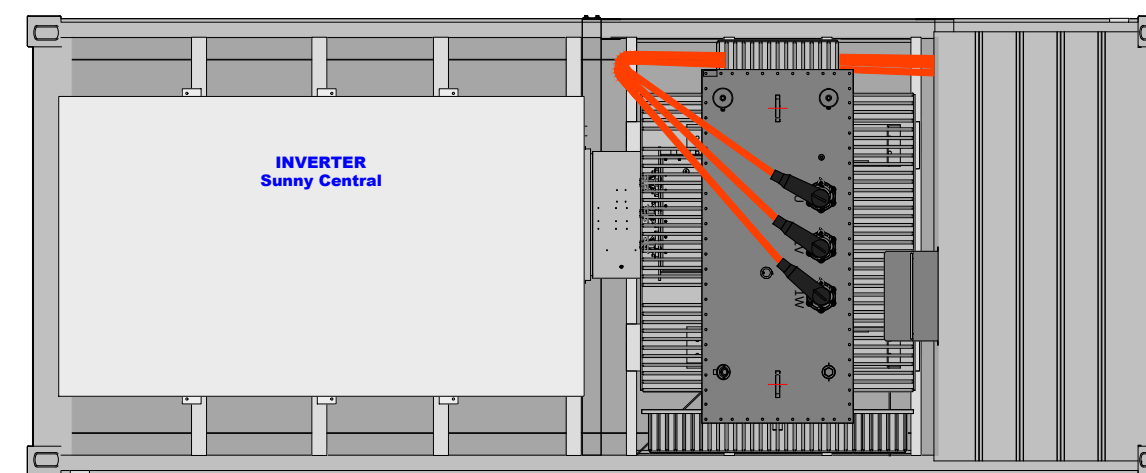
VISTA DALL'ALTO
