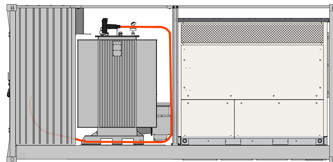
LATO SINISTRO
